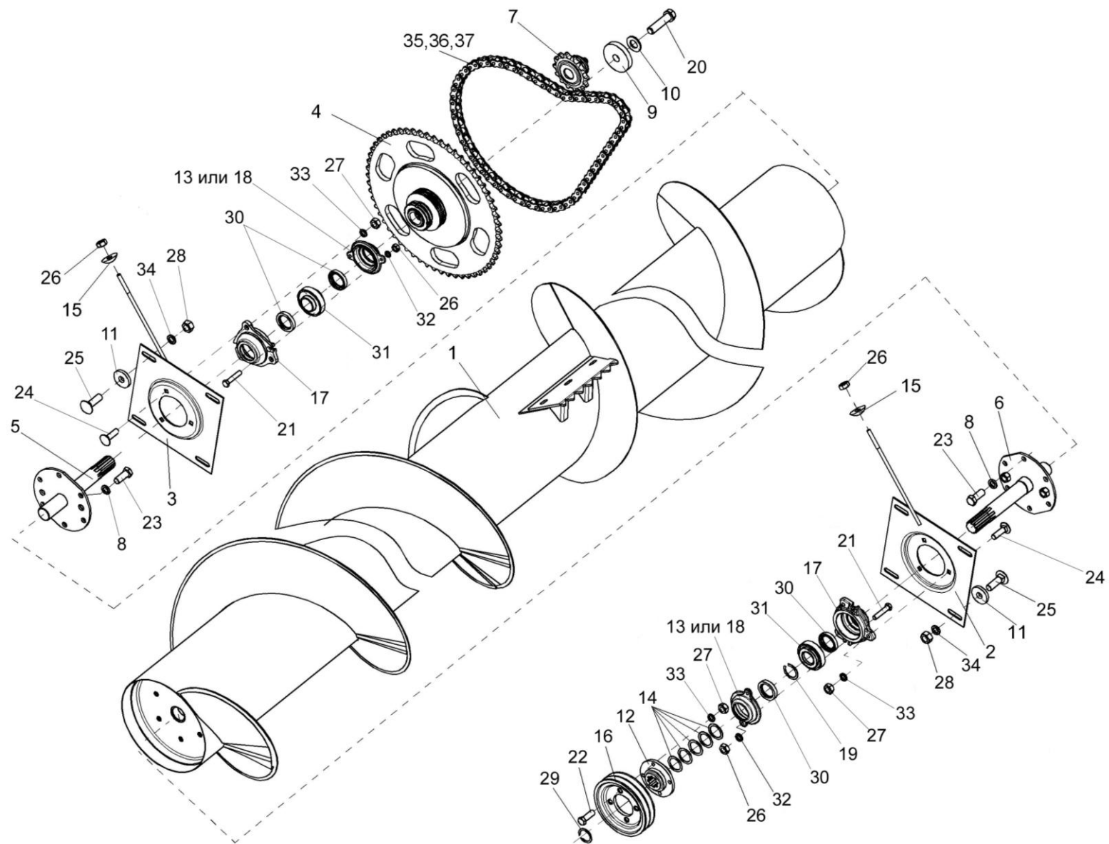
Рисунок 59 - Установка шнека
