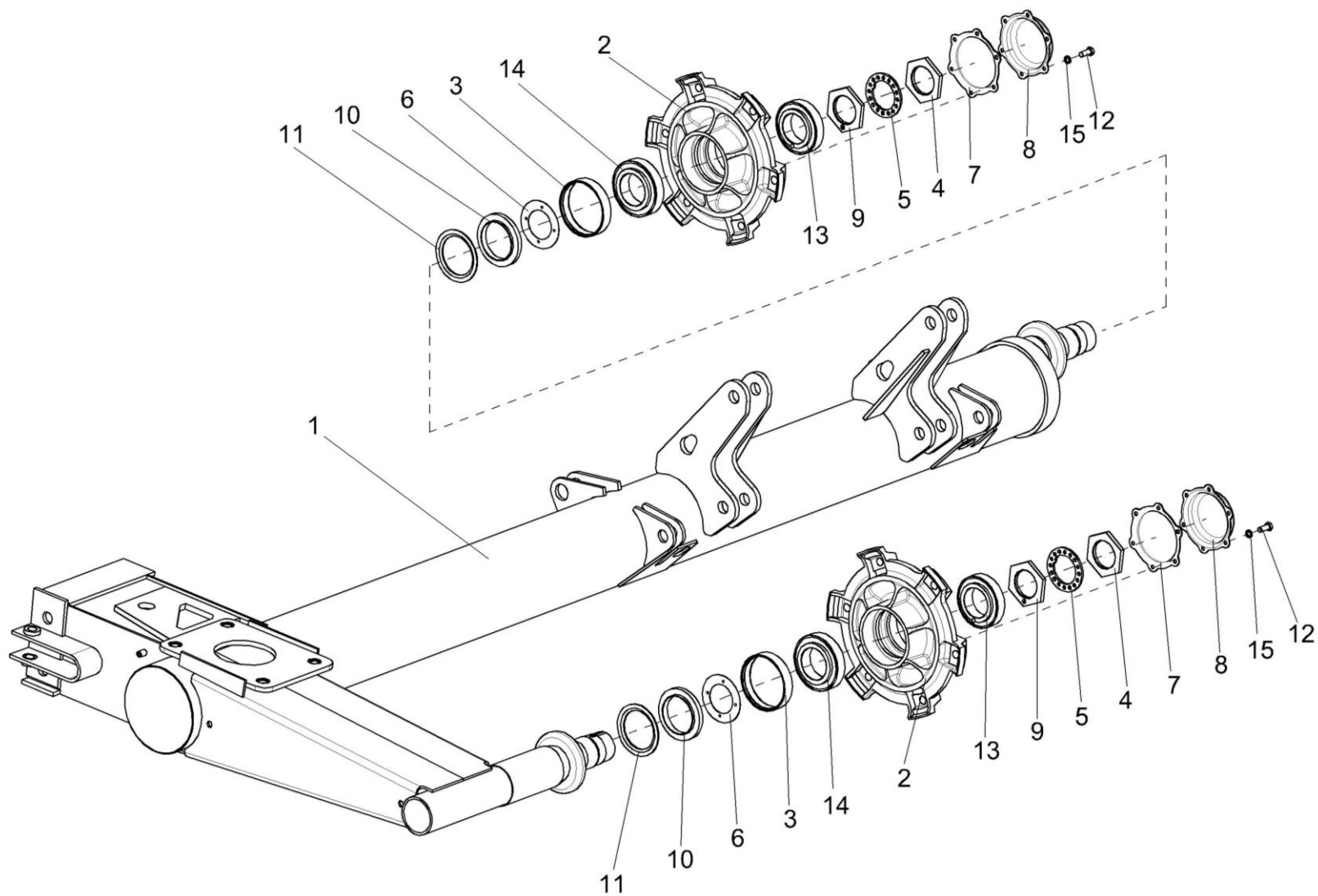
Рисунок 5 – Рама со ступицами КПТ 0100100
