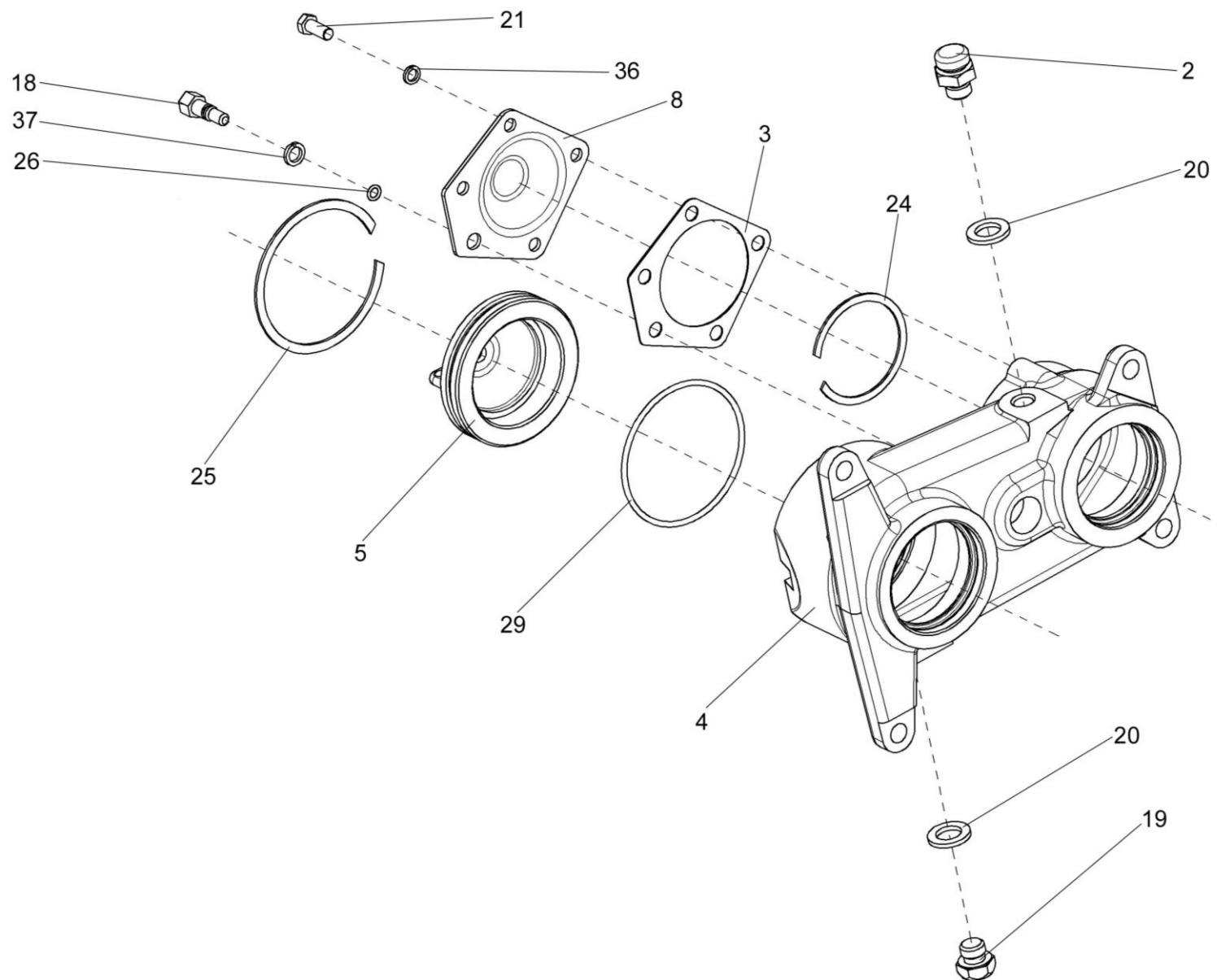
Рисунок 39 – Редуктор нижних вальцев ПКК 0117000А (лист 1)
