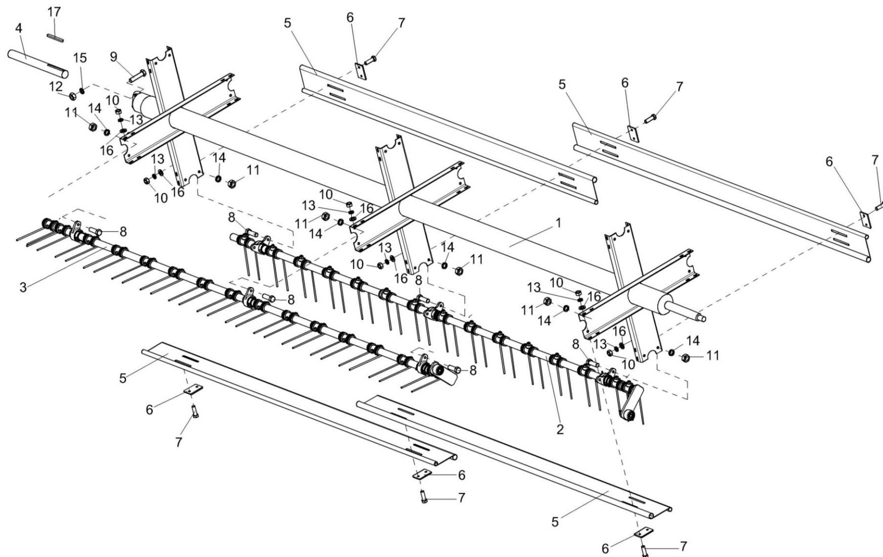
Рисунок 64 - Мотовило (установка граблин)
