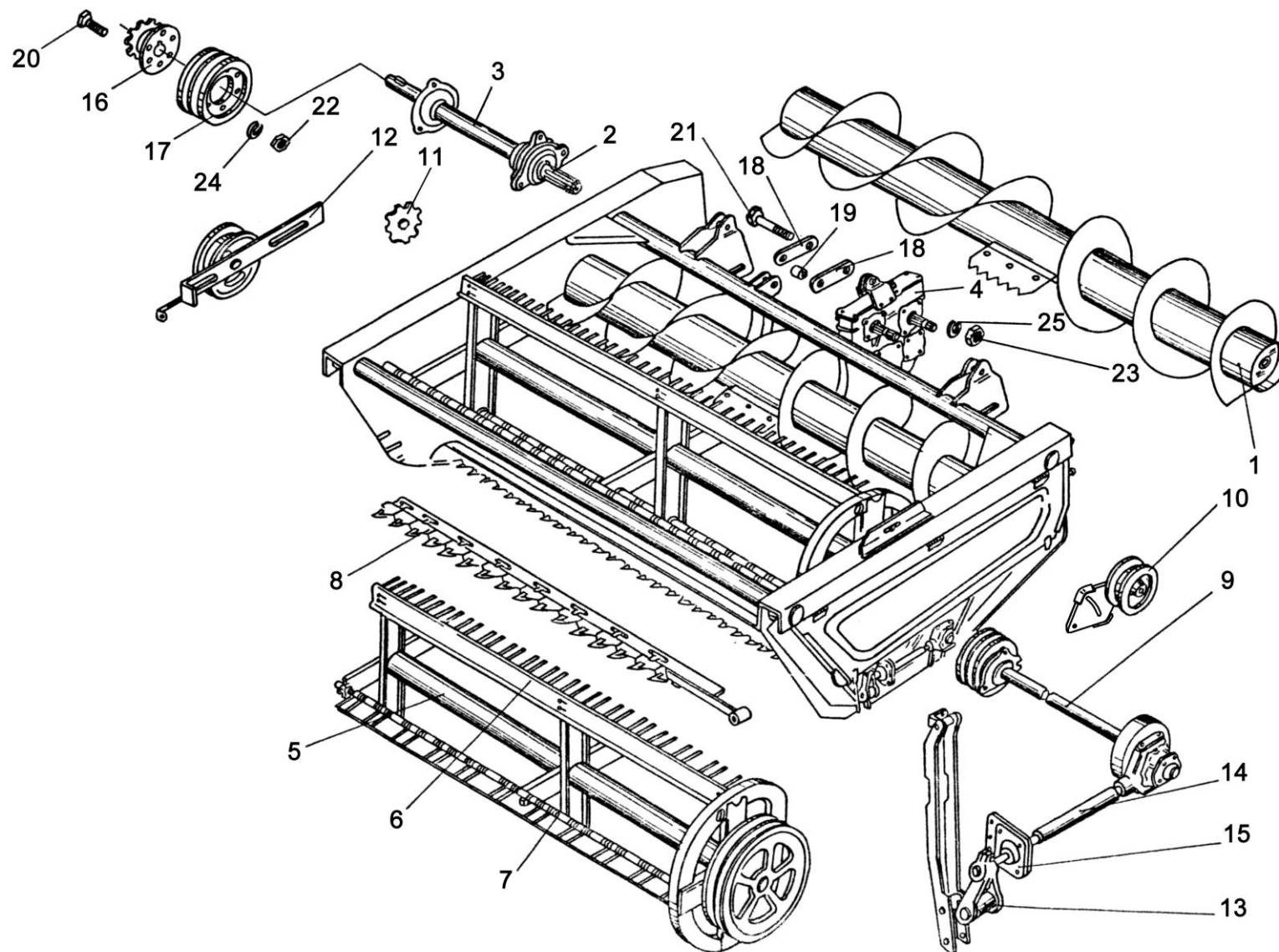
Рисунок 57 - Жатка для уборки трав. Общий вид КПТ 0460000
