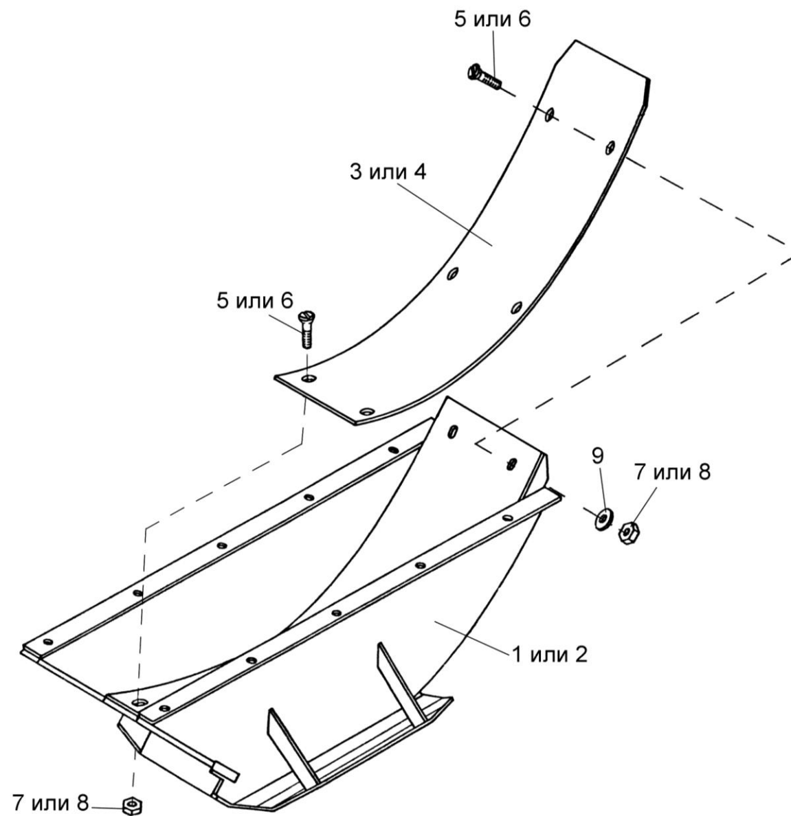
Рисунок 20 – Кожух нижний ПКК 0102000А
