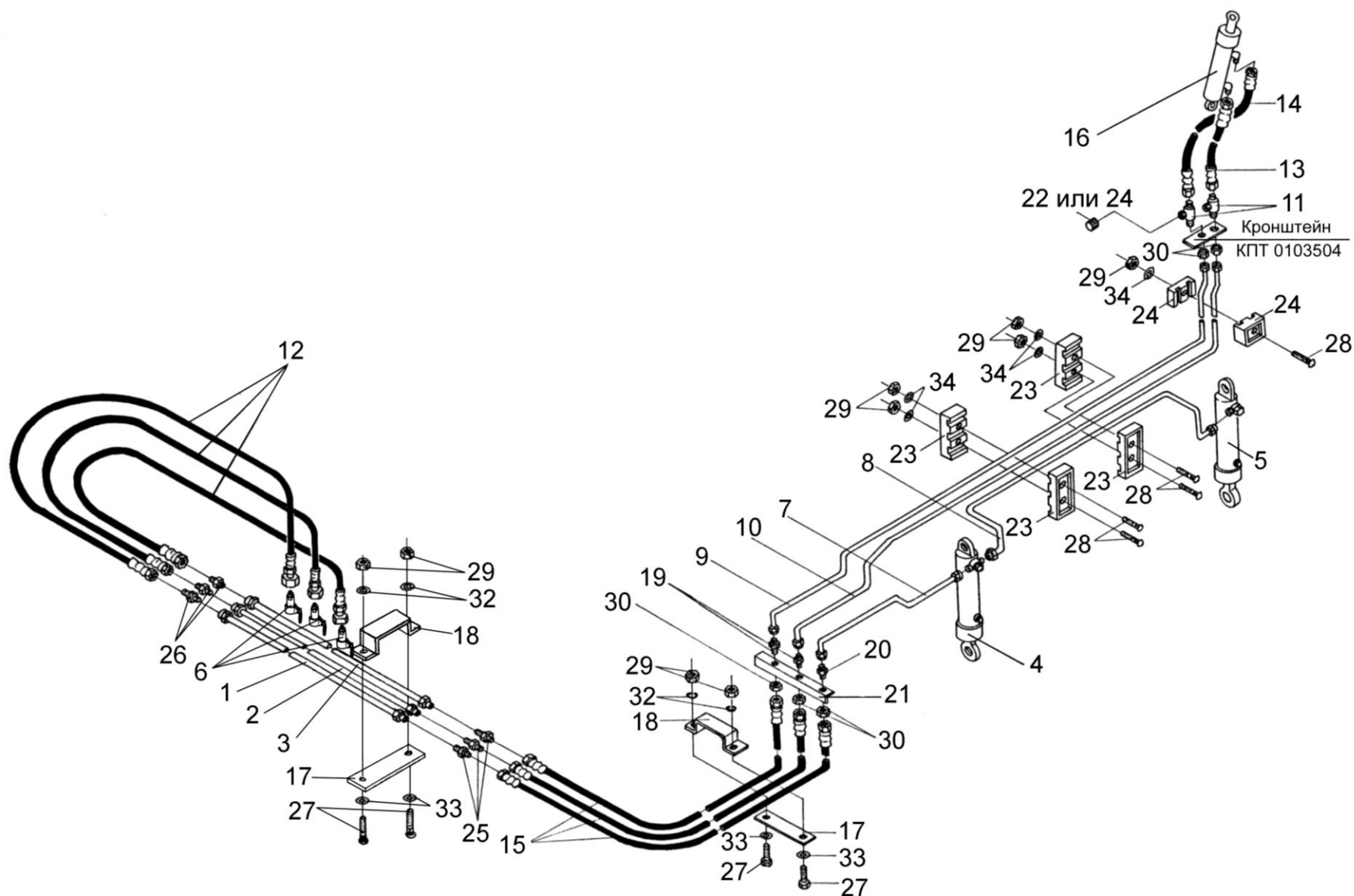
Рисунок 15 – Гидросистема прицепа
