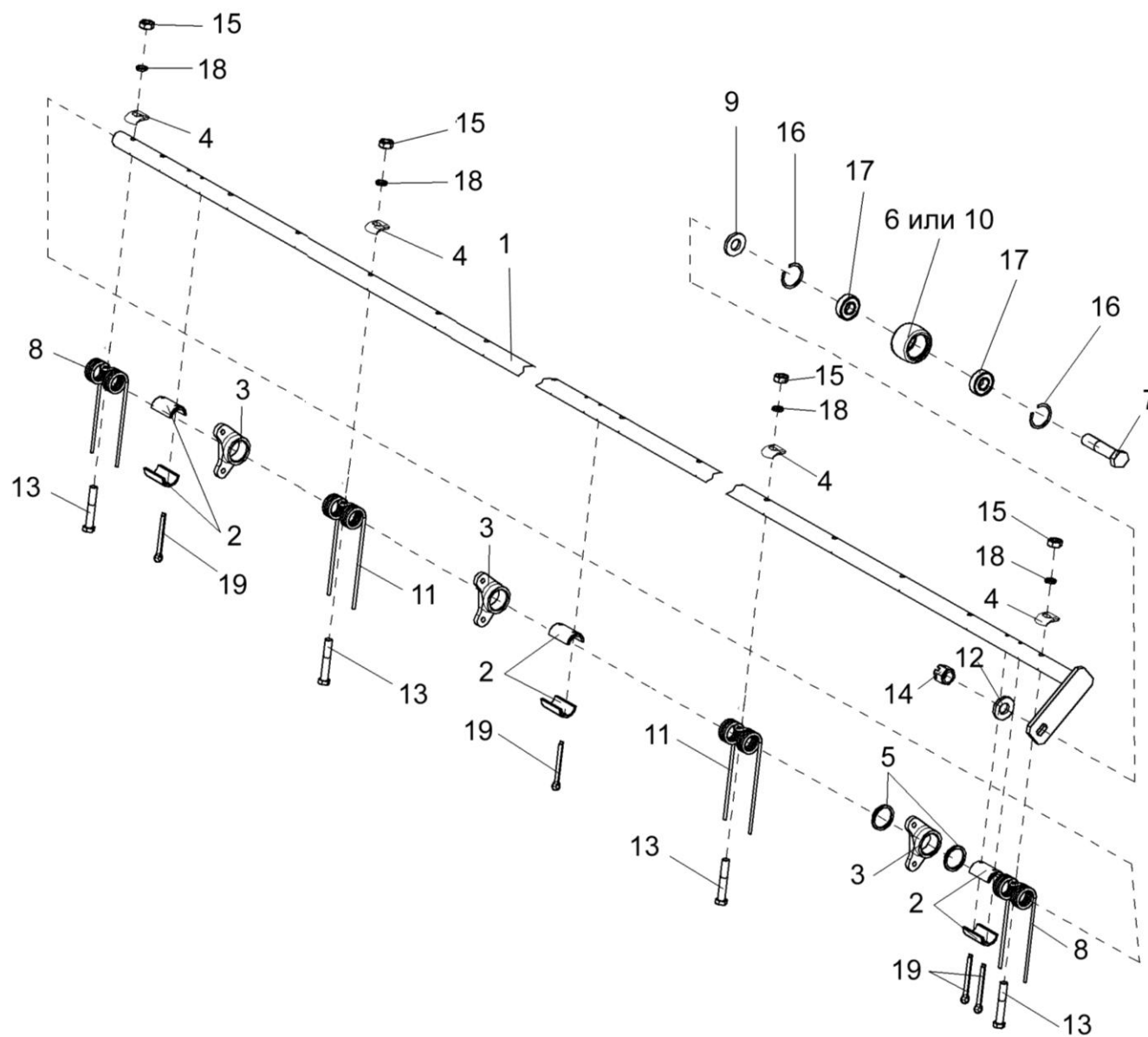
Рисунок 67 - Граблина КИН 0203030
