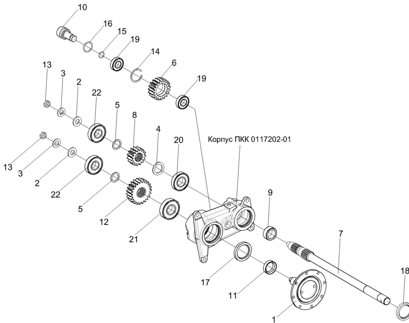
Рисунок 18 – Редуктор нижних вальцев ПКК 0117000А-01 (лист 2)
