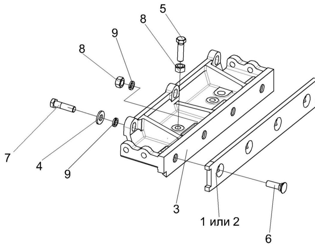
Рисунок 9 – Противорез ПКК 0100170
