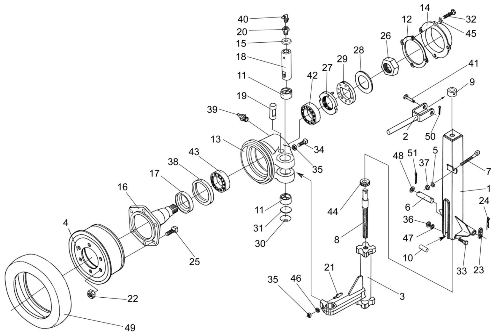
Рисунок 12 – Колесо опорное ПКК 0143000
