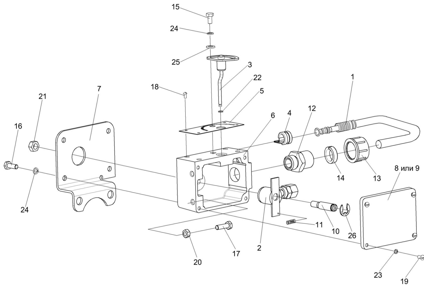
Рисунок 21 – Датчик камнедетектора ПКК 0108320Б
