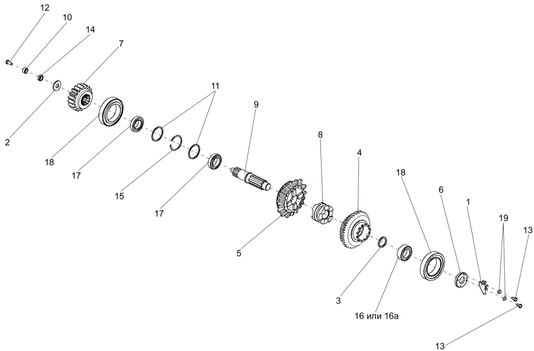
Рисунок 26 – Вал ПКК 0135040А
