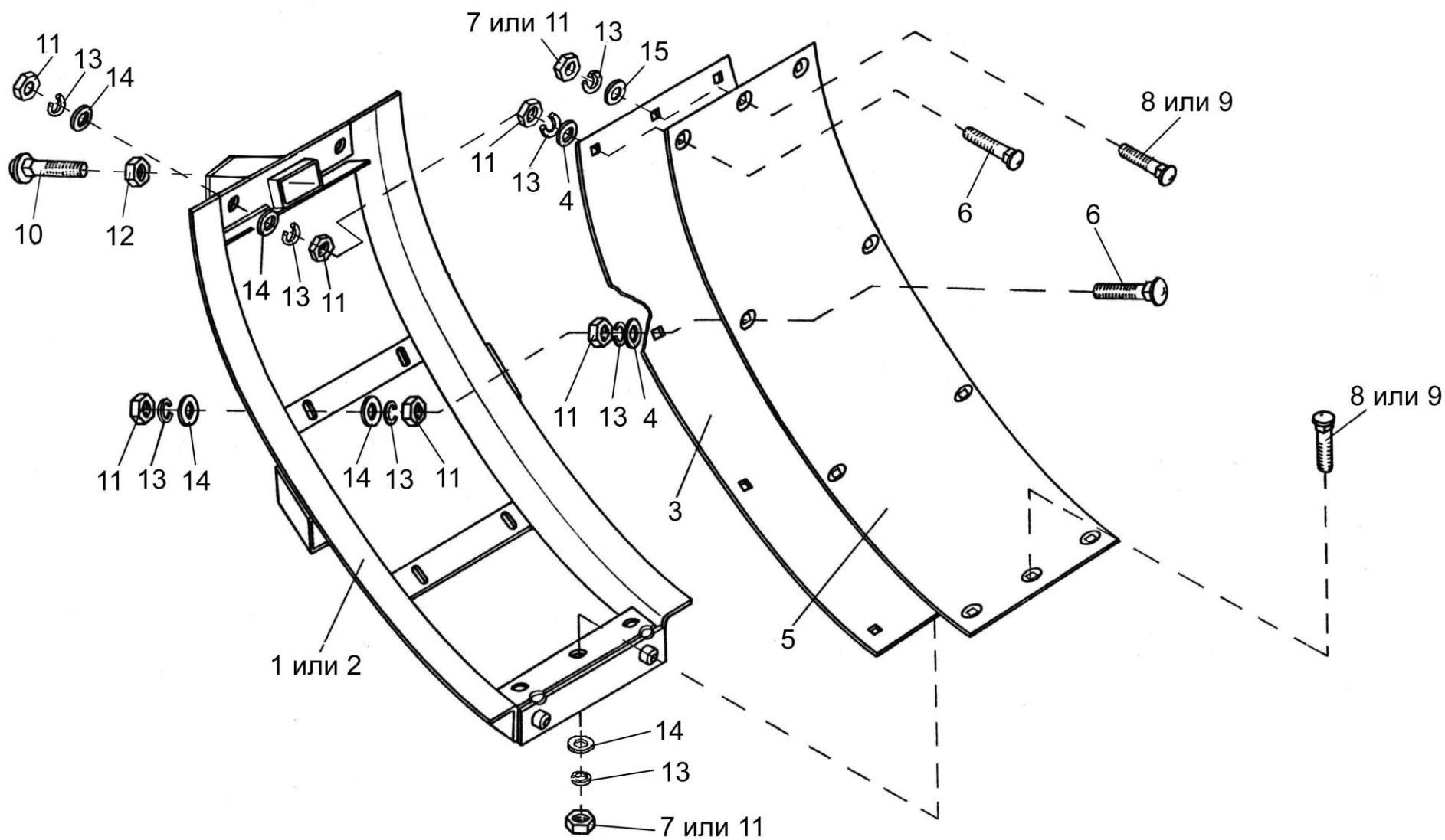
Рисунок 5 – Терка ПКК 0138000Б
