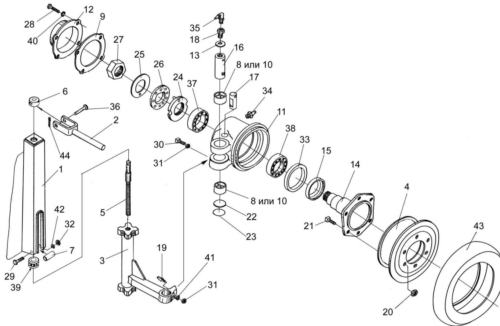
Рисунок 13 – Колесо опорное ПКК 0144000-01
