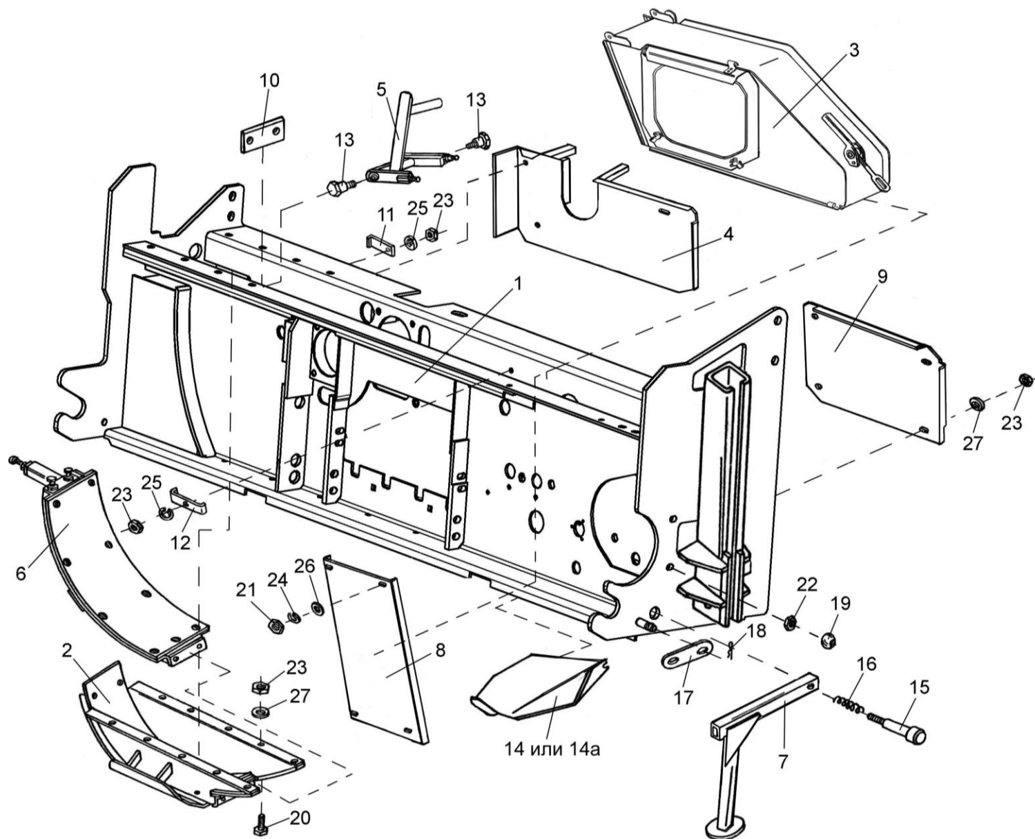
Рисунок 3 – Рама измельчителя ПКК 0101000А
