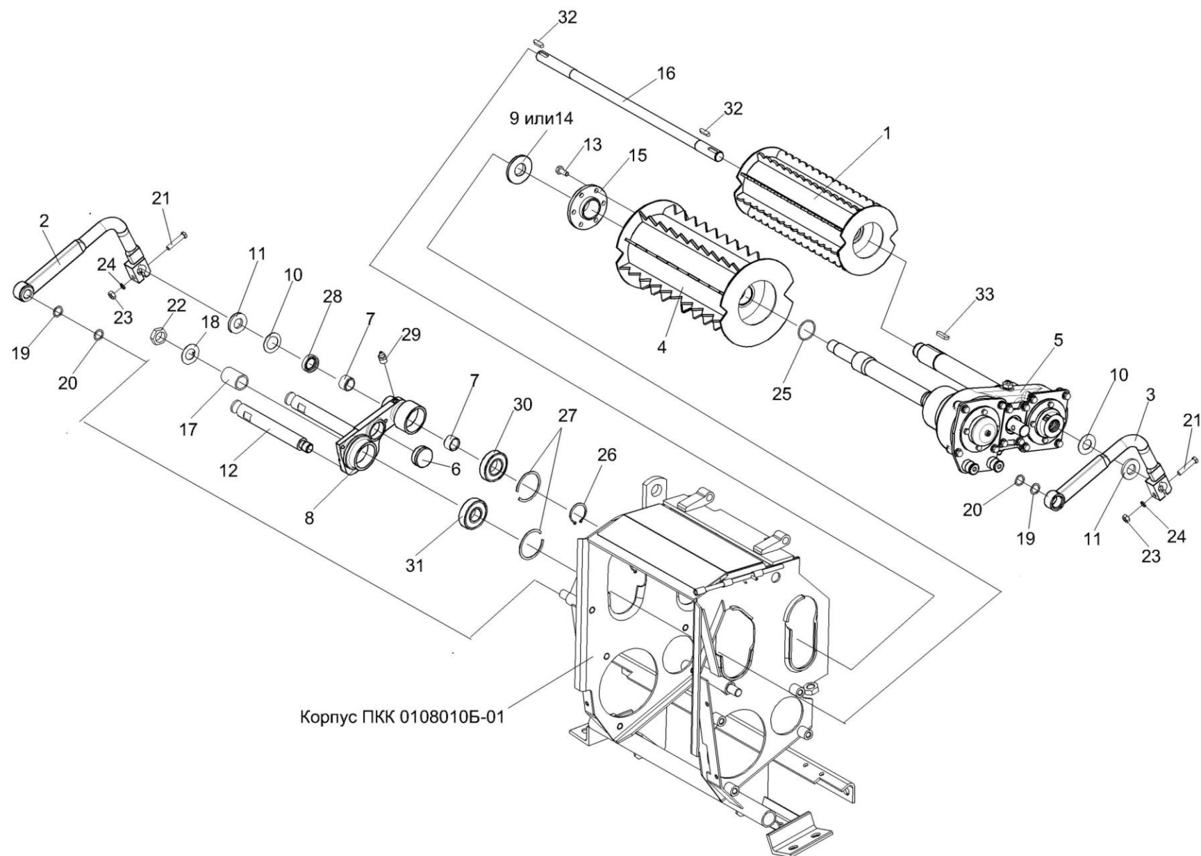
Рисунок 16 – Аппарат питающий ПКК 0108000Б (установка редуктора ПКК 0118000Б-01)
