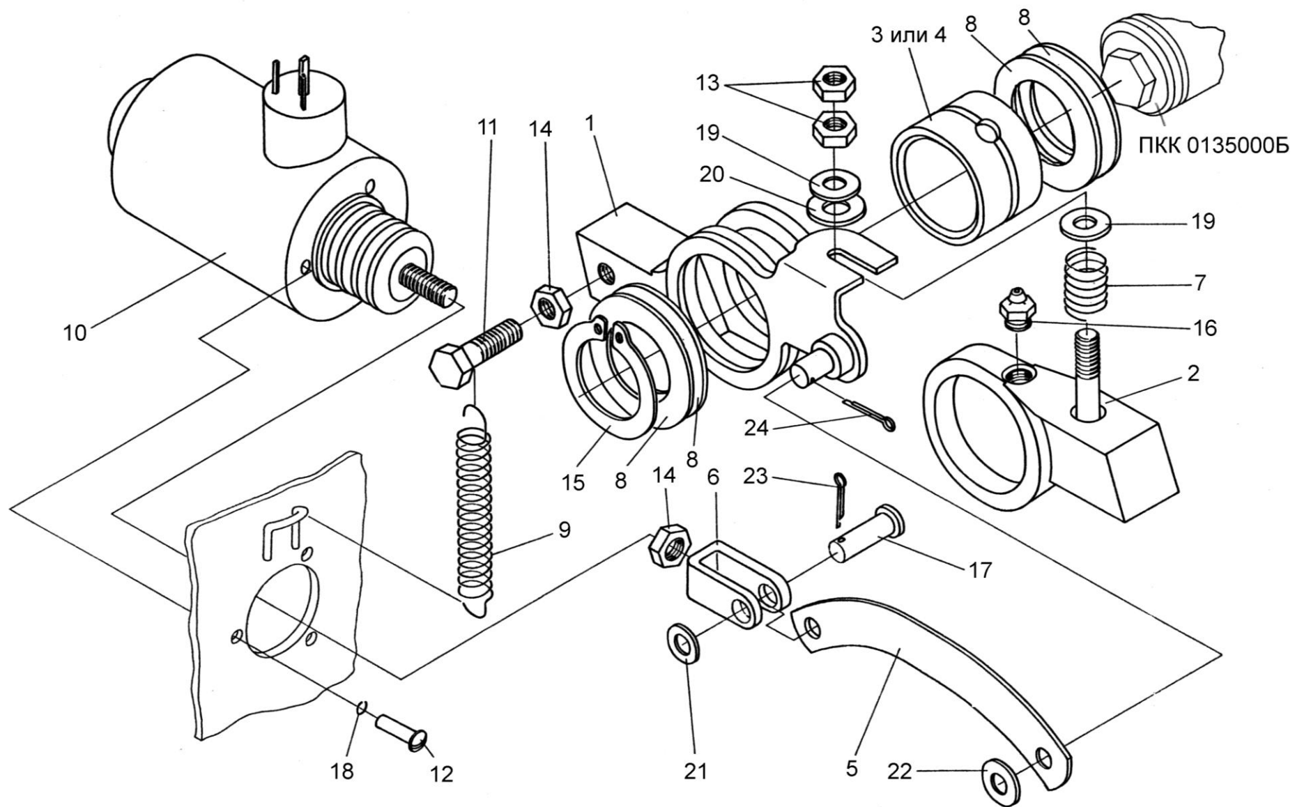
Рисунок 33 – Механизм быстрого останова
