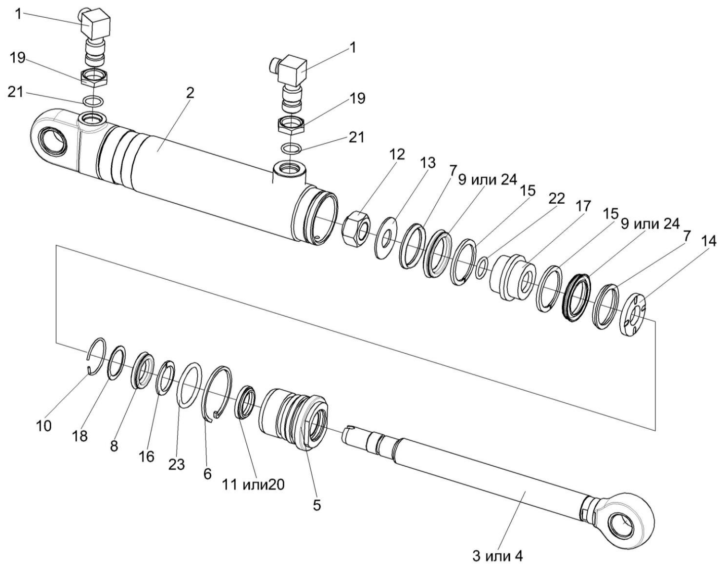
Рисунок 47 – Гидроцилиндр ПКК 0113200
