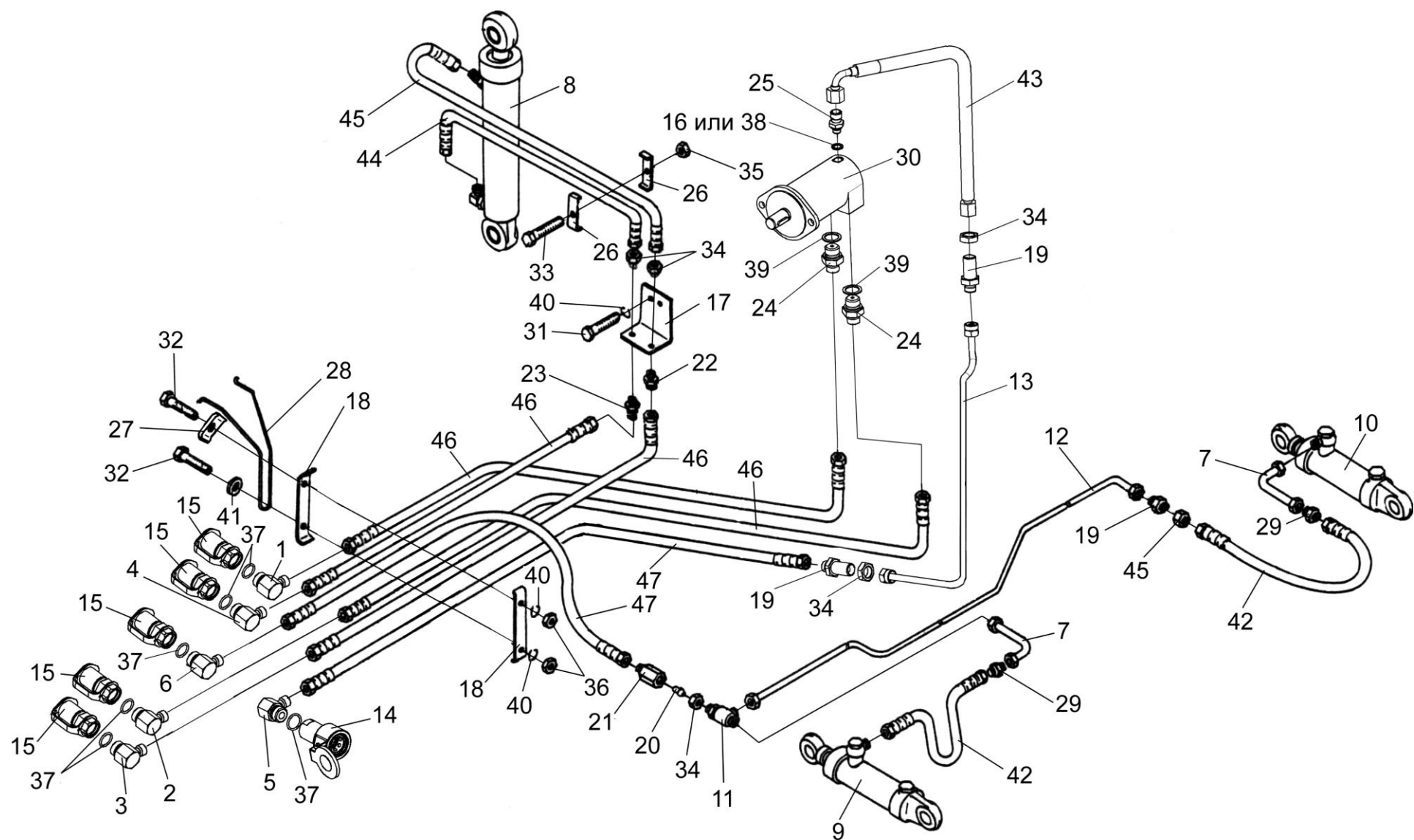
Рисунок 46 – Гидросистема полунавесного комбайна ПКК 0113000А
