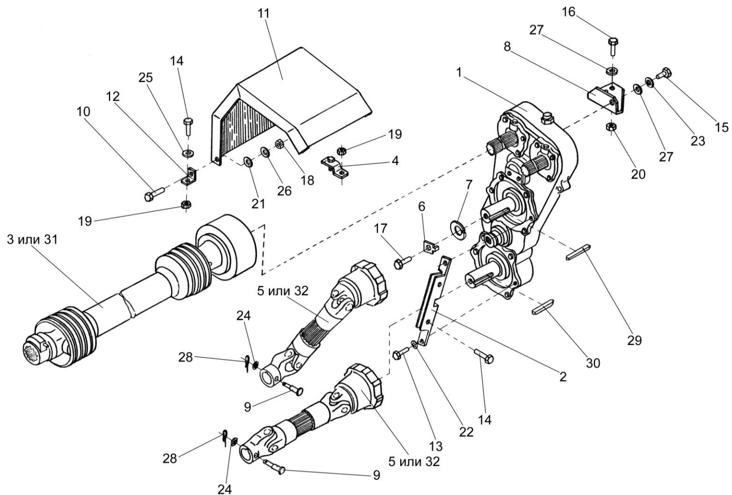
Рисунок 30 – Установка валов карданных ПКК 0140000 и ПКК 0145000
