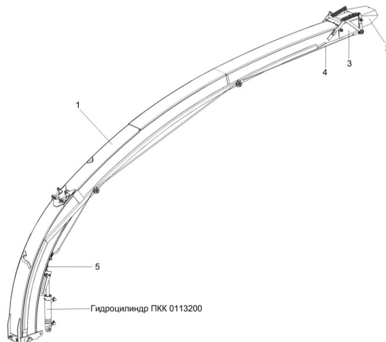
Рисунок 39 – Силосопровод PKK 0109000B
