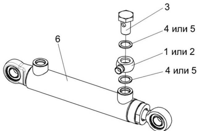
Рисунок 48 – Гидроцилиндр ПКК 0113210
