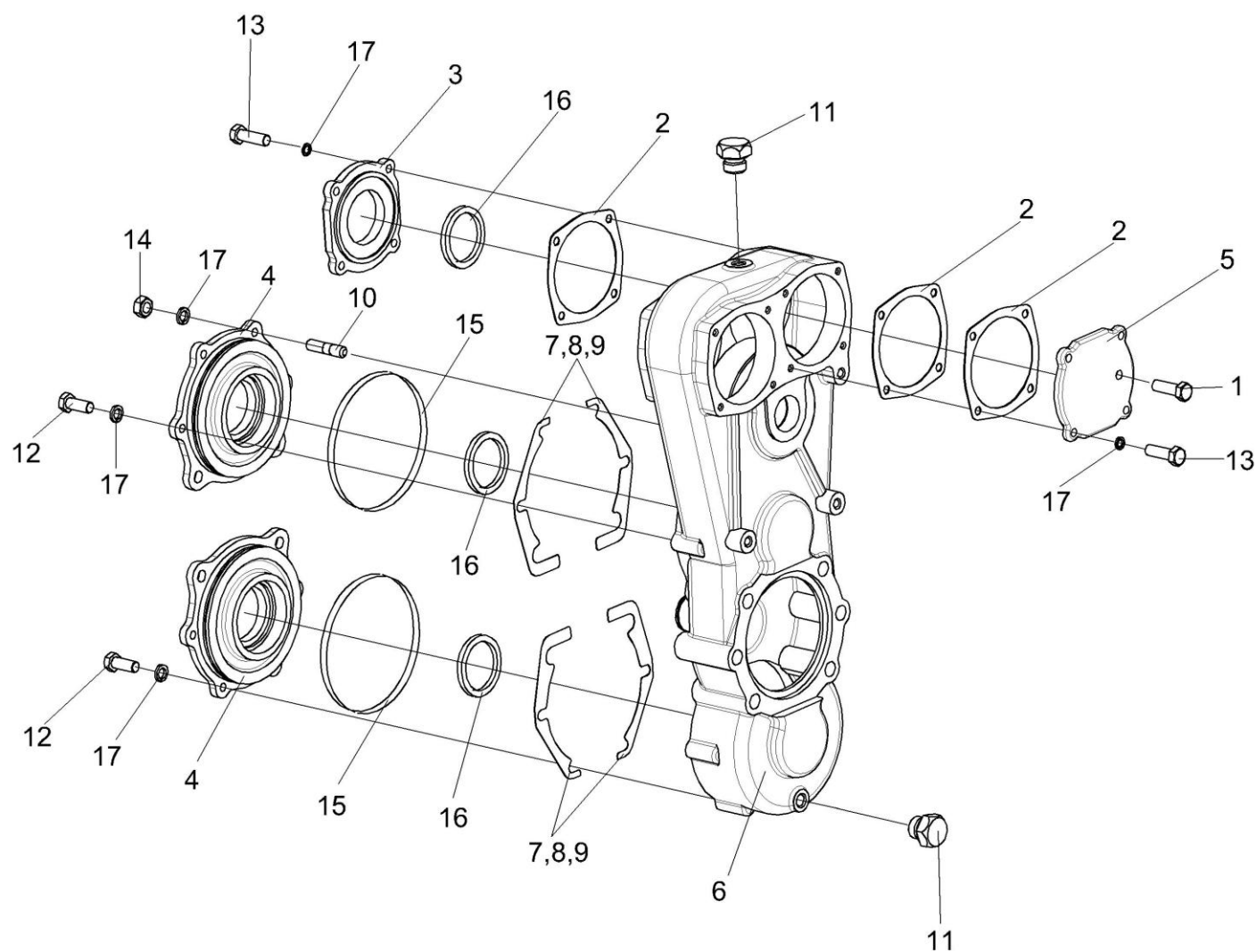
Рисунок 28 – Редуктор цилиндрический ПКК 0135170 (корпус и крышки)
