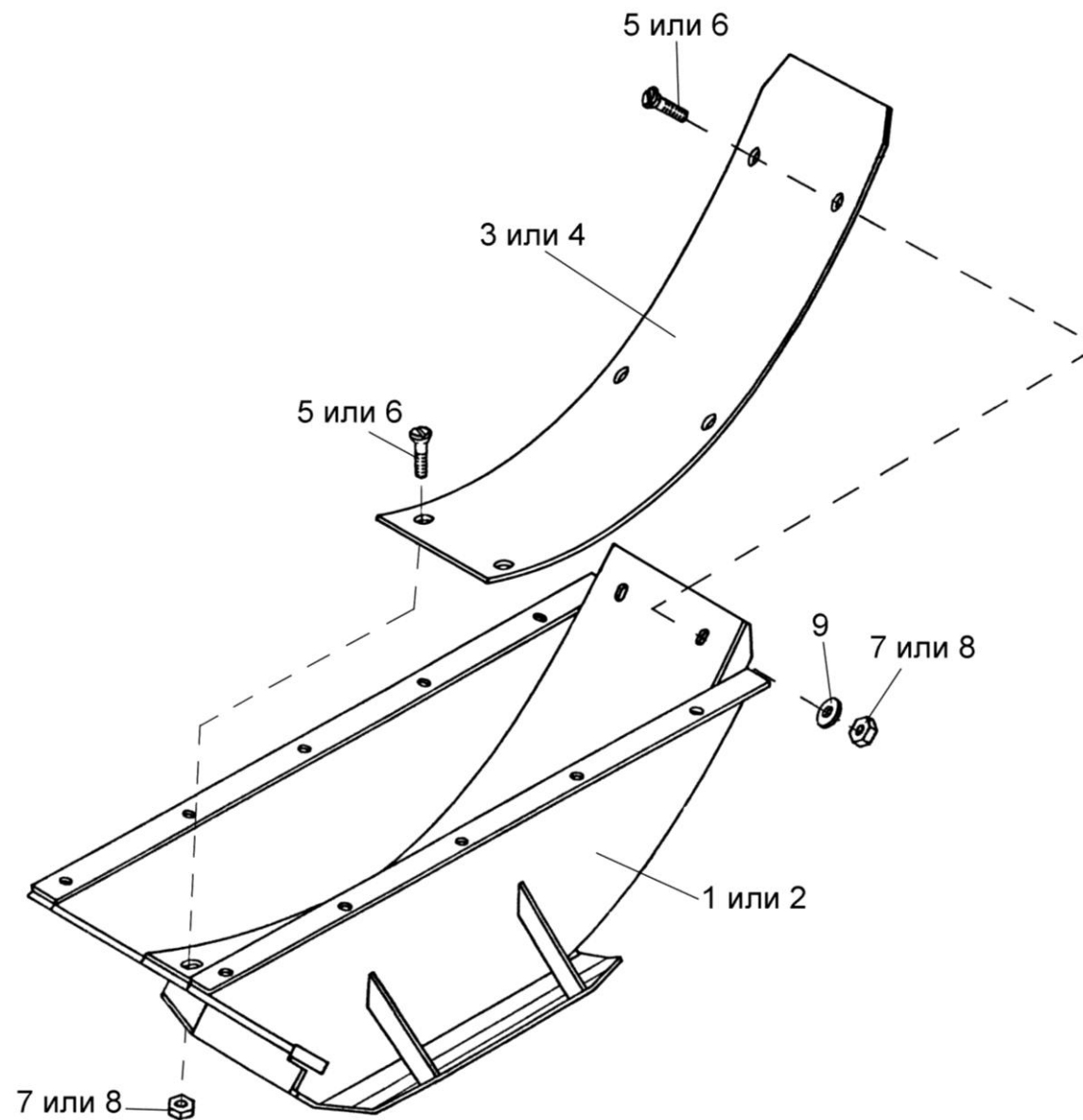
Рисунок 4 – Кожух нижний ПКК 0102000А
