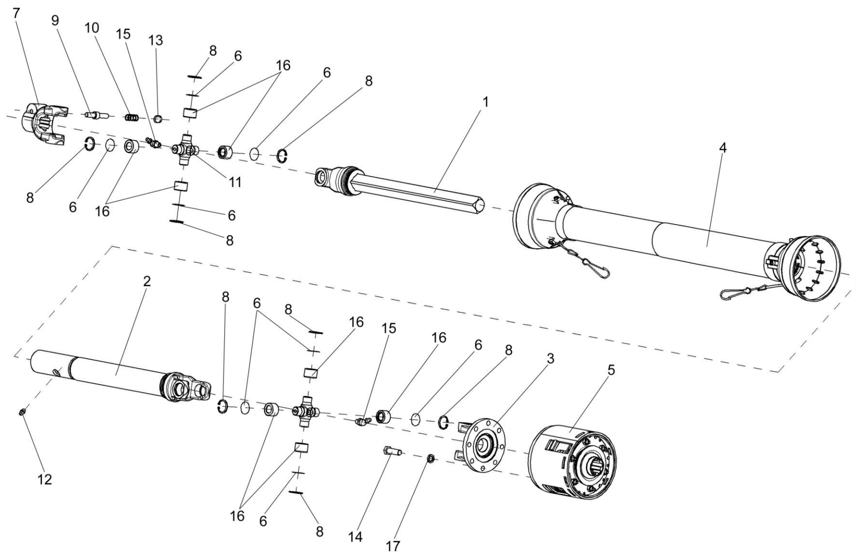
Рисунок 31 – Вал карданный телескопический с защитным кожухом ПКК 0140000
