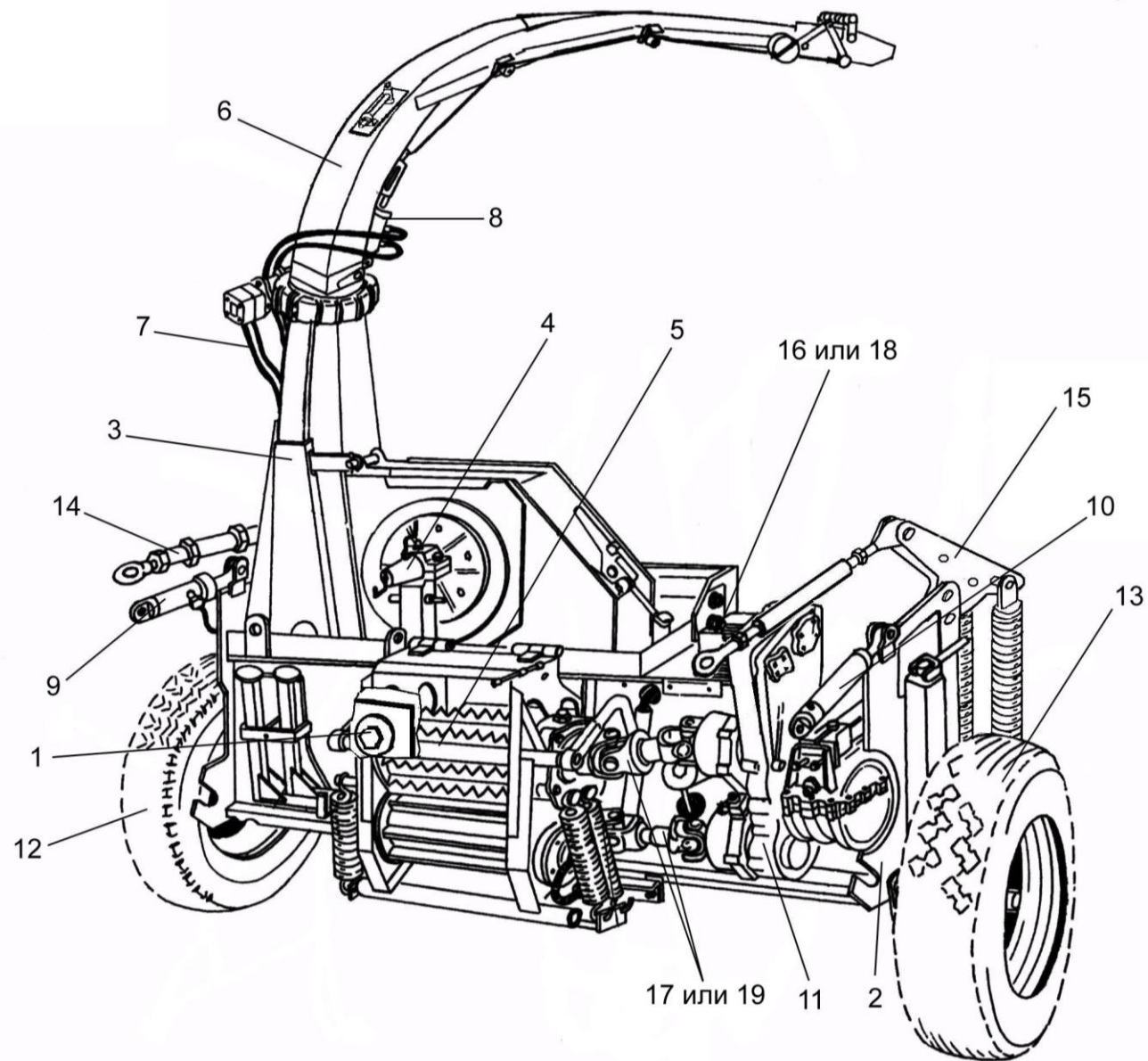
Рисунок 2 – Измельчитель ПКК 0100000А
