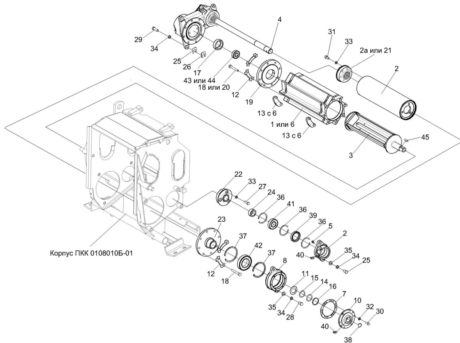
Рисунок 15 – Аппарат питающий ПКК 0108000Б (установка редуктора нижних валцов ПКК 0117000А-01)
