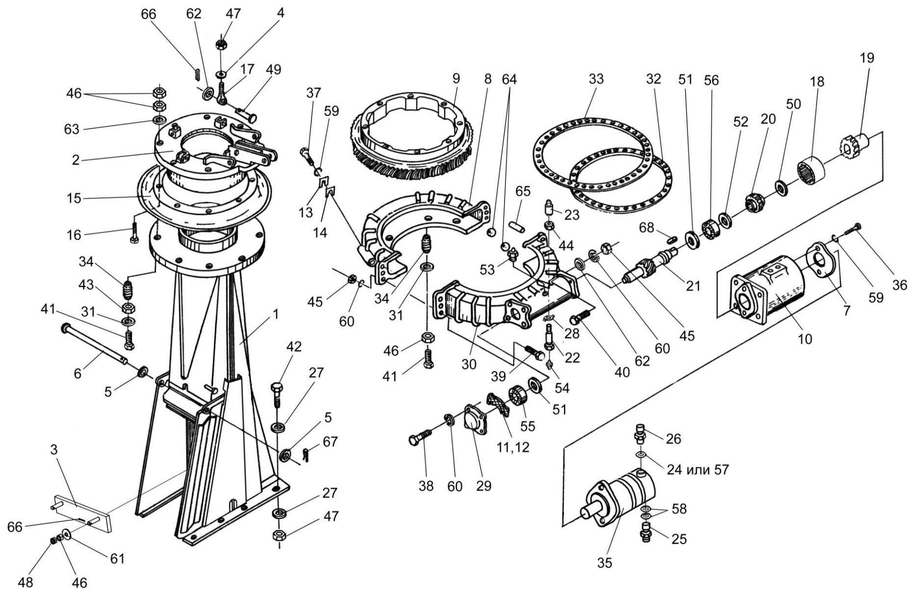
Рисунок 38 – Основание силосопровода ПКК 0104030А
