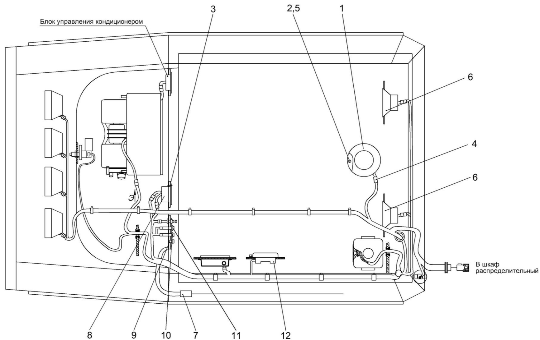
Рисунок 92 – Электрооборудование кабины КГС 0120000 (вид сверху)
