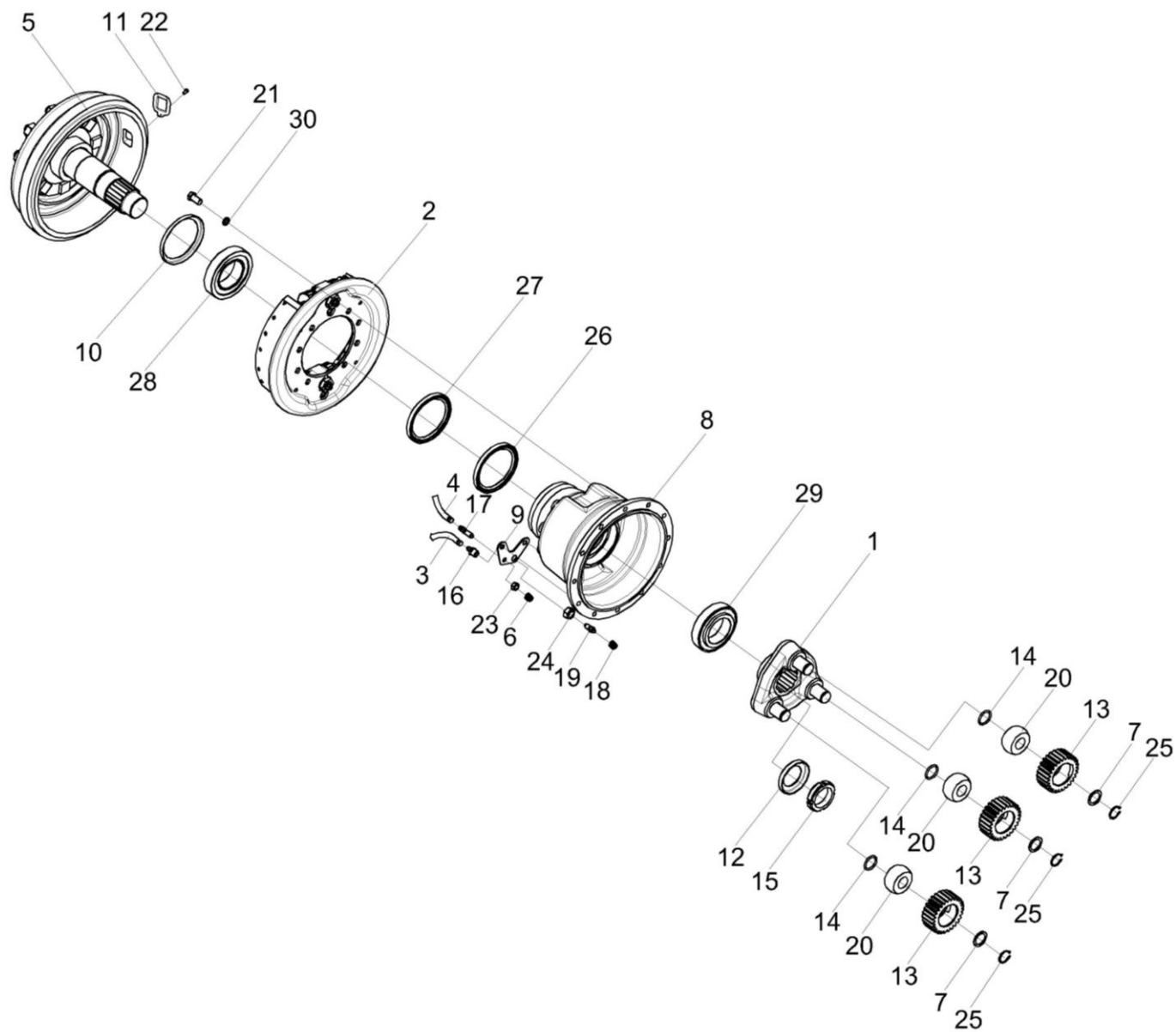
Рисунок 71 – Редуктор бортовой 54-4-4
