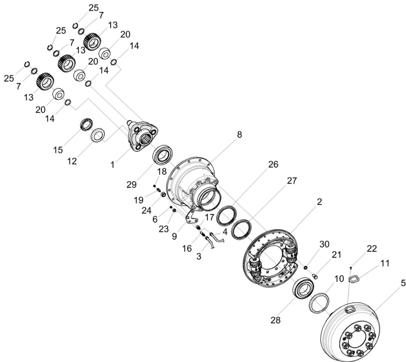
Рисунок 70 – Редуктор бортовой 54-4-3
