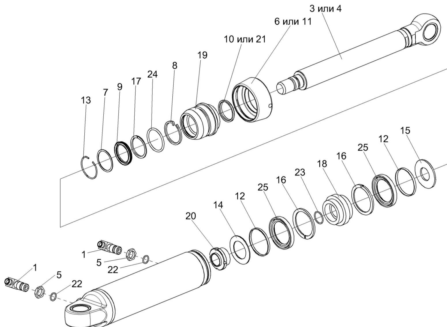
Рисунок 159 – Гидроцилиндр КИЛ 0118440-02
