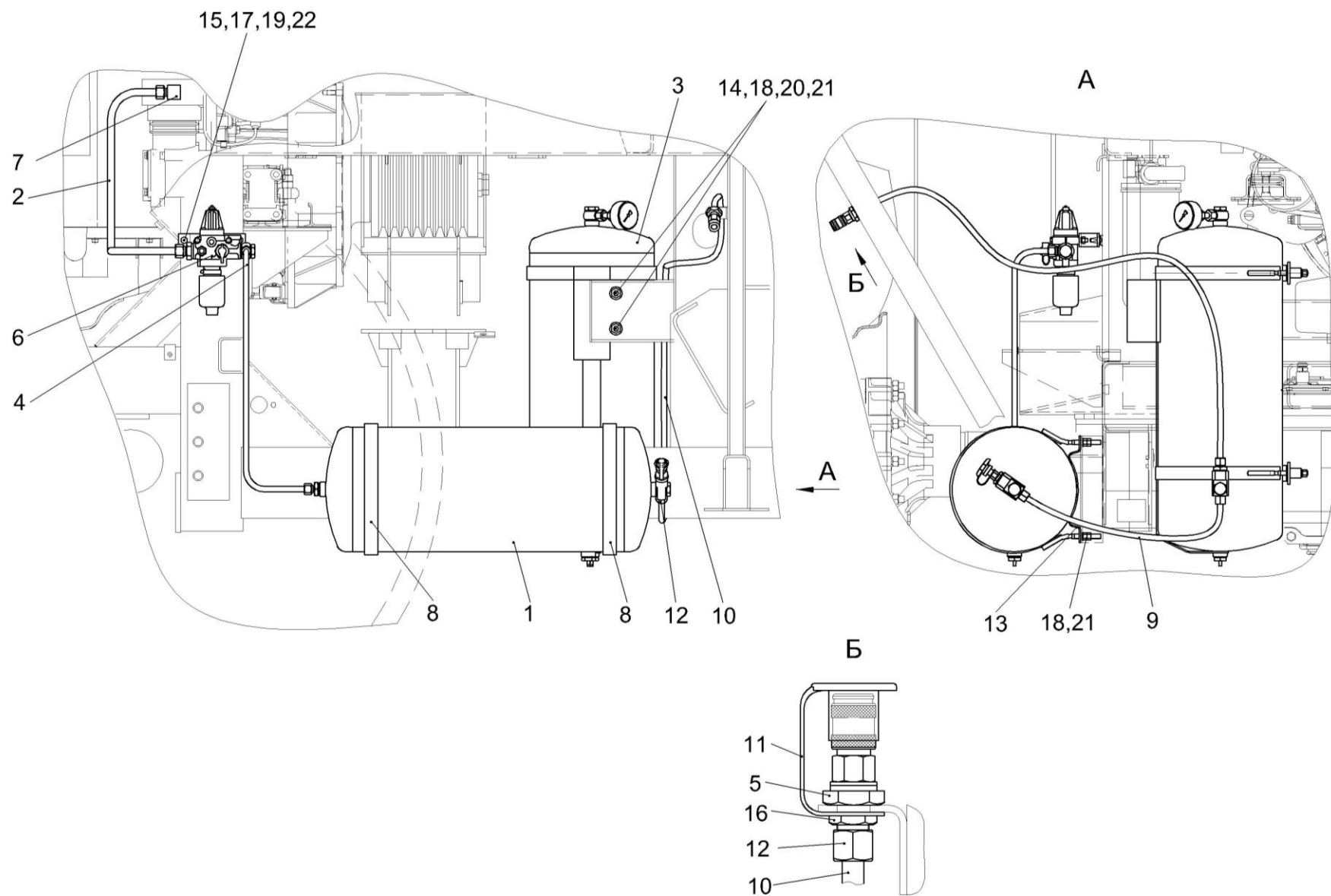
Рисунок 160 – Пневмосистема КГС 0180000
