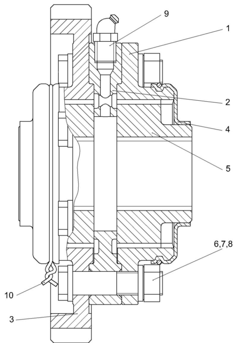
Рисунок 57 – Муфта КЗК-10-0107150
