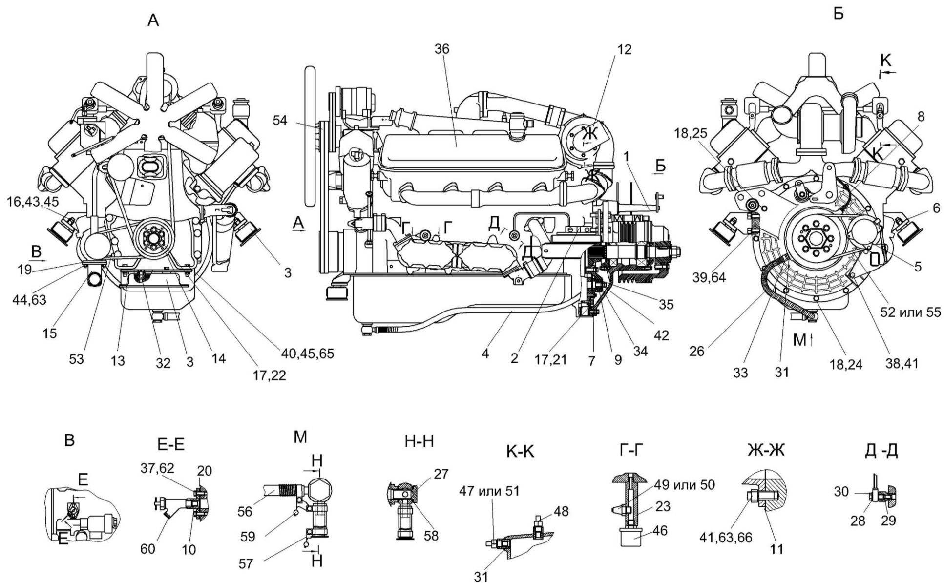
Рисунок 5 – Двигатель КЗК-10-0106010
