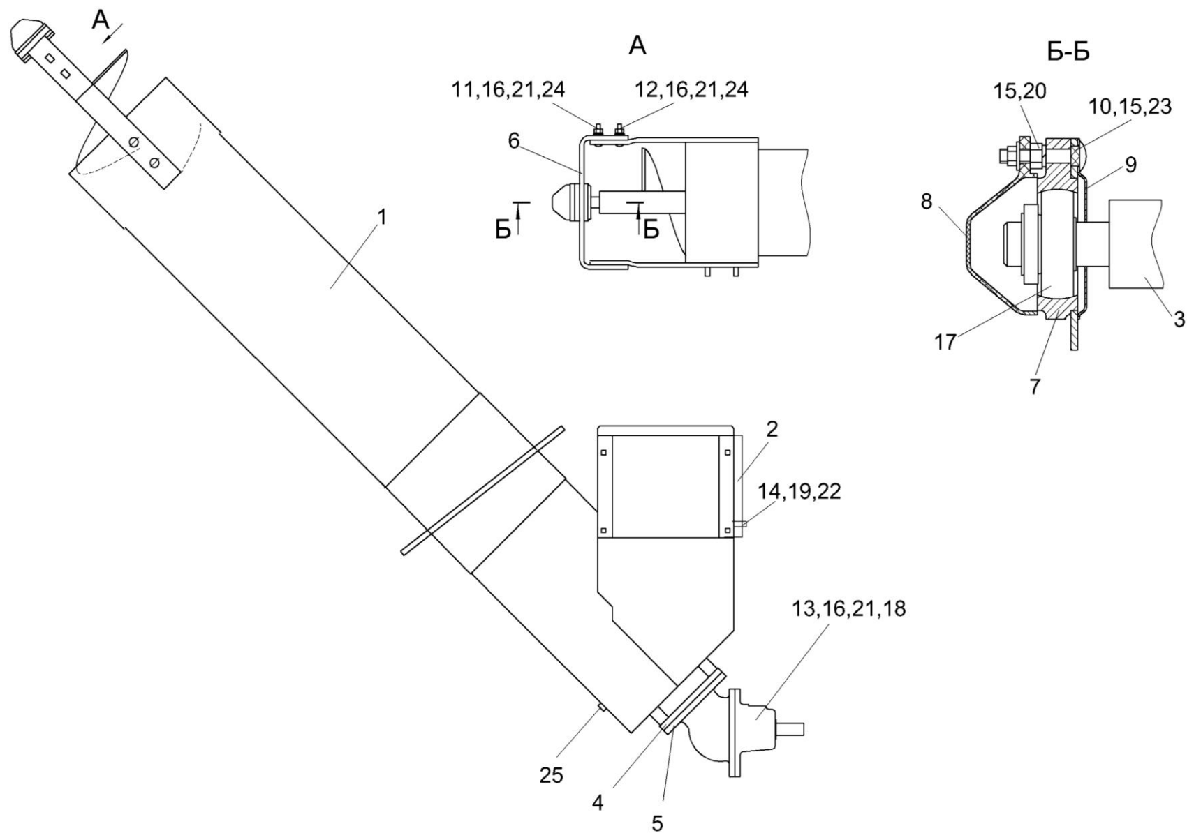
Рисунок 70 – Шнек загрузной зерновой КЗК-10-0216000
