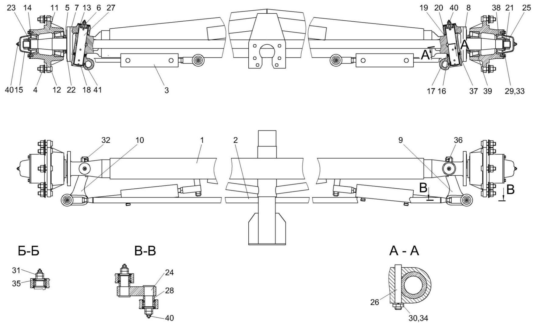
Рисунок 58— Мост управляемых колес КЗК-10-0109000
