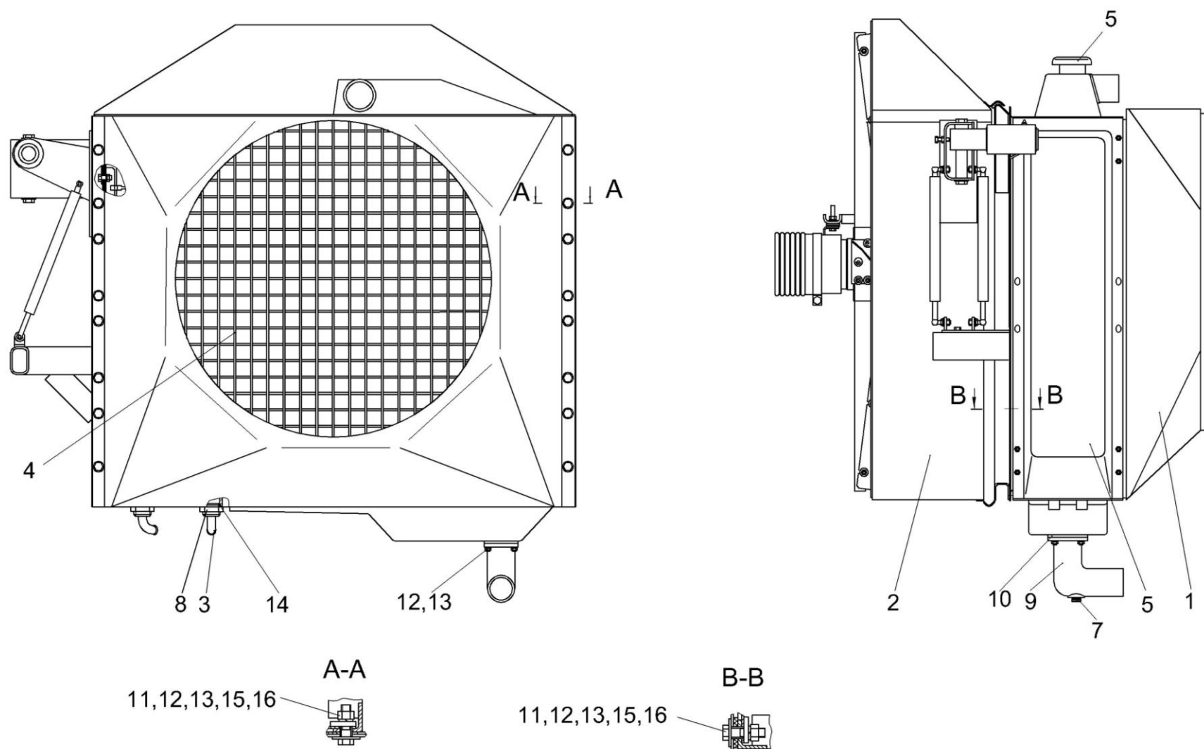
Рисунок 8 – Радиатор КЗК-10-0106040
