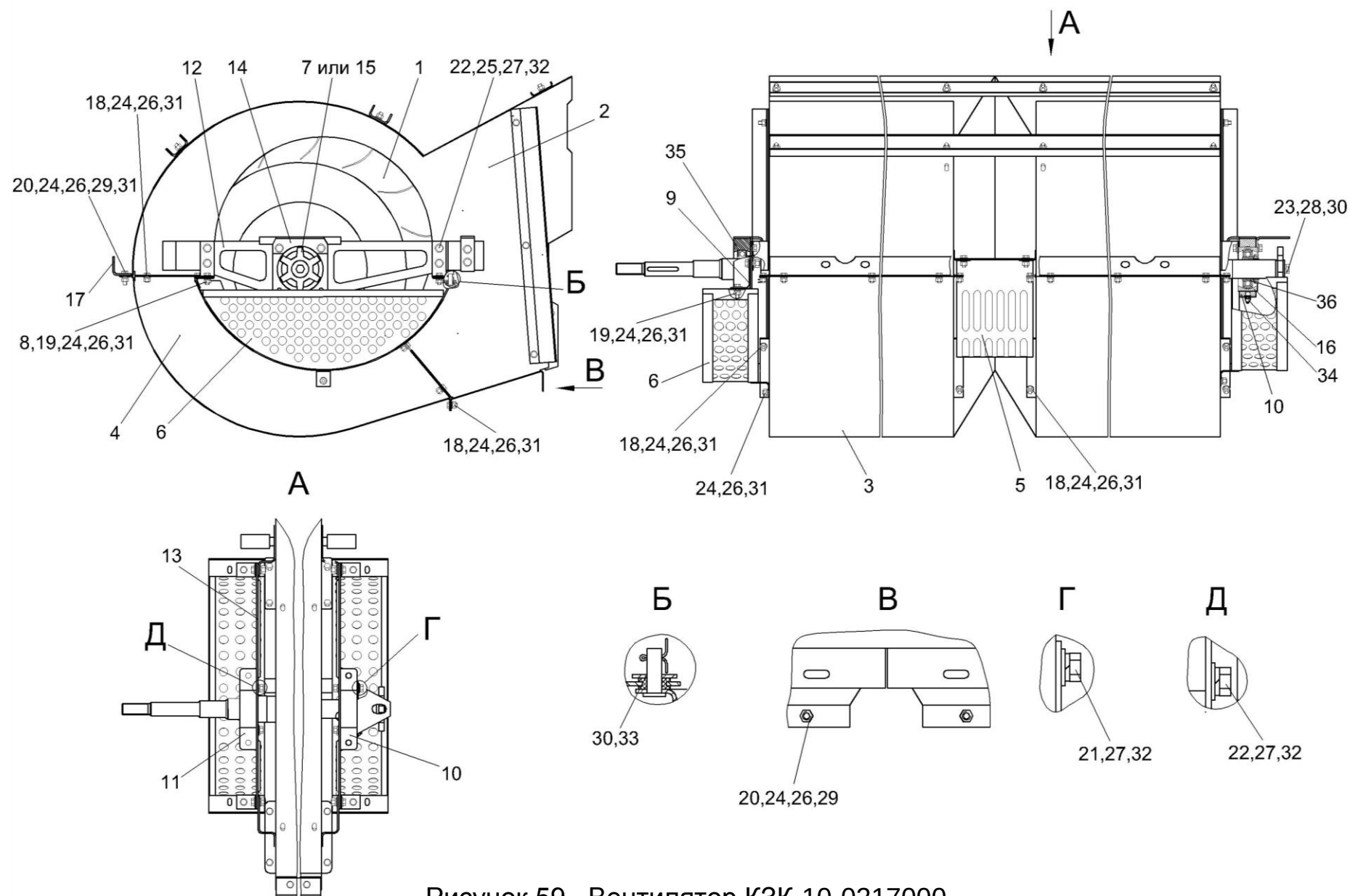
Рисунок 59– Вентилятор КЗК-10-0217000
