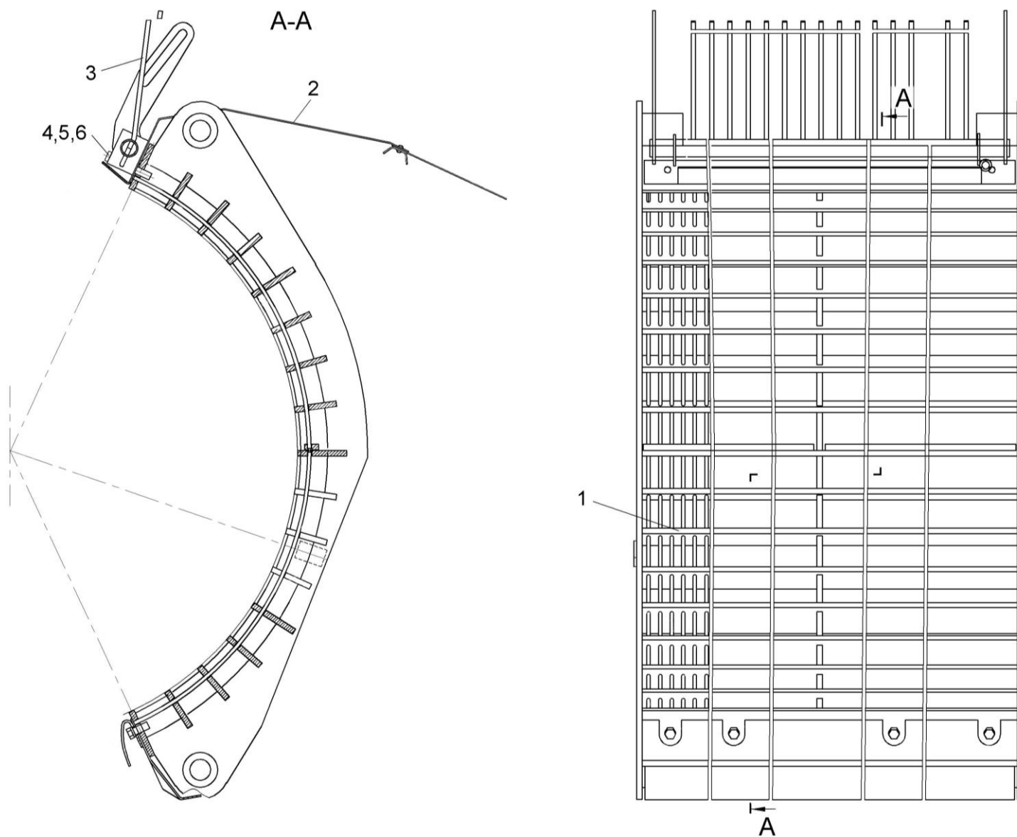
Рисунок 50 – Подбарабанье КЗК-10-0103000
