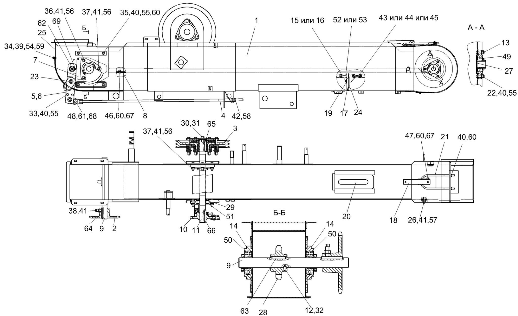
Рисунок 68 – Элеватор зерновой КЗК-10-0214000
