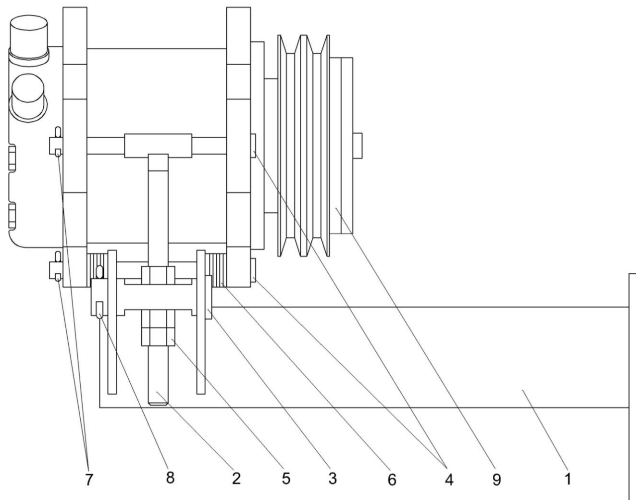
Рисунок 7 – Компрессор K3K-10-0113050
