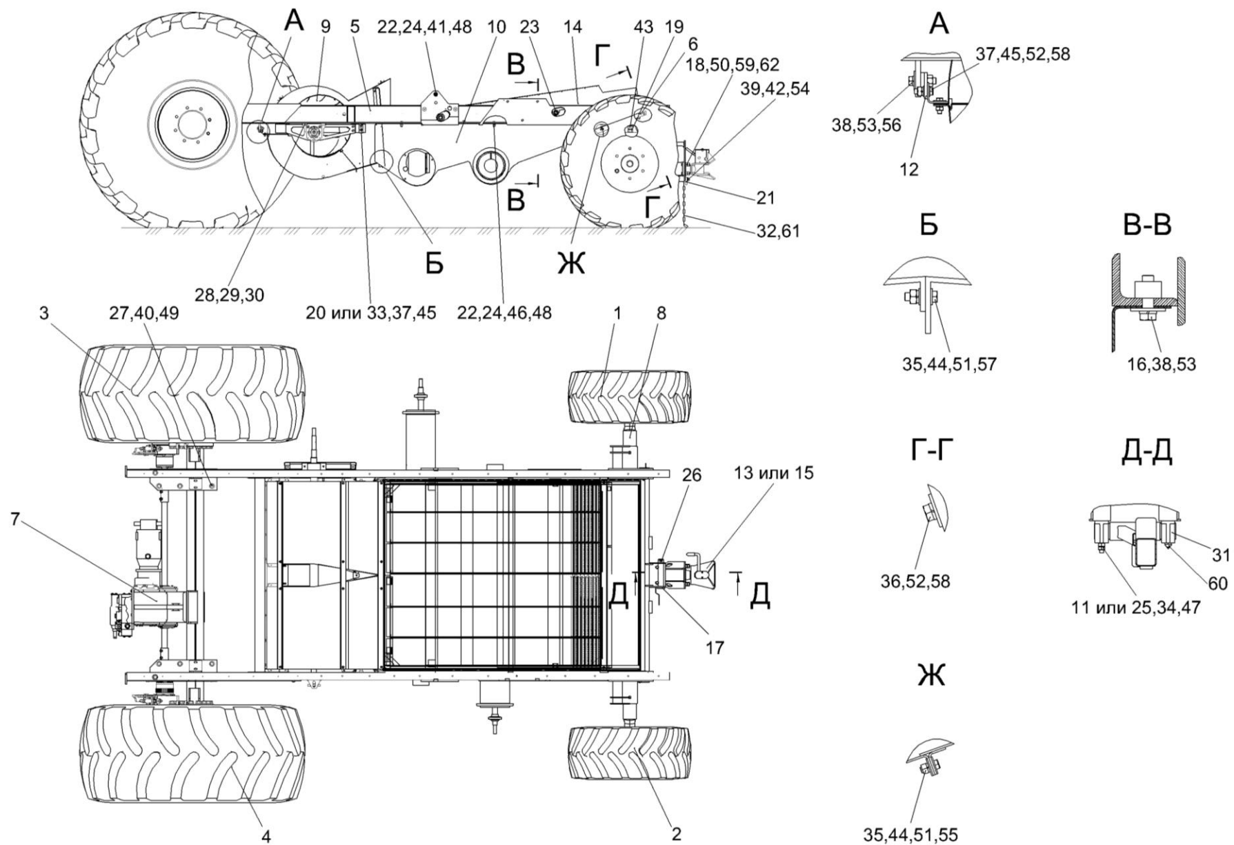
Рисунок 54 – Шасси КЗК-10-0111000
