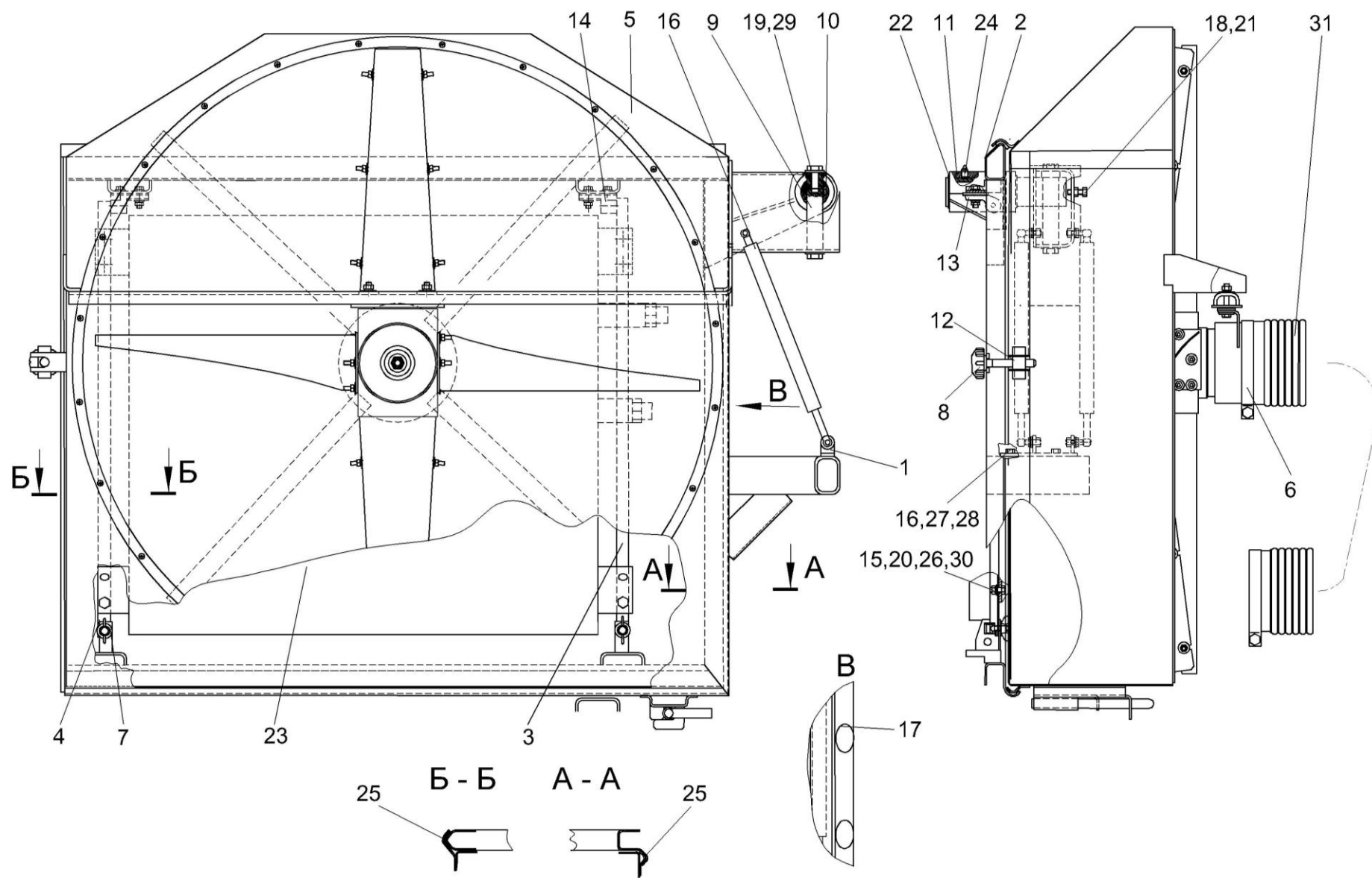
Рисунок 9 – Воздухозаборник КЗК-10-0112000
