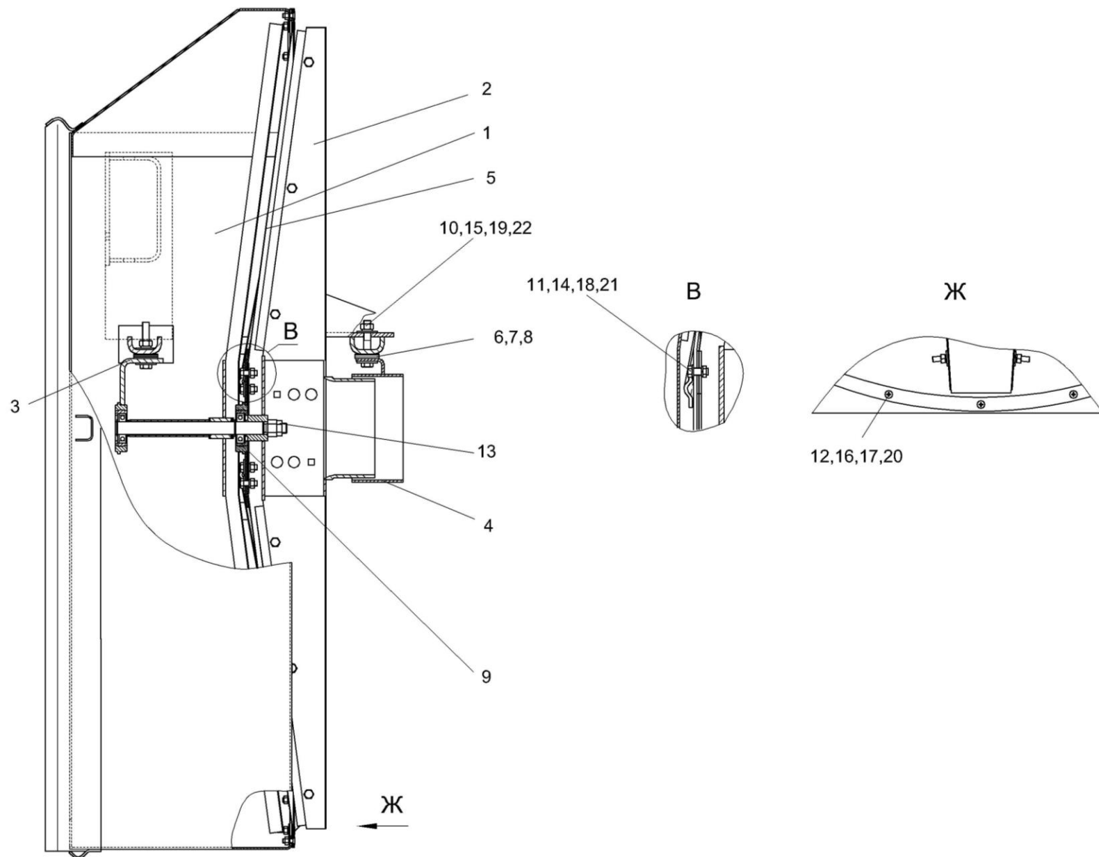
Рисунок 10 – Воздухозаборник КЗК-10-0112190
