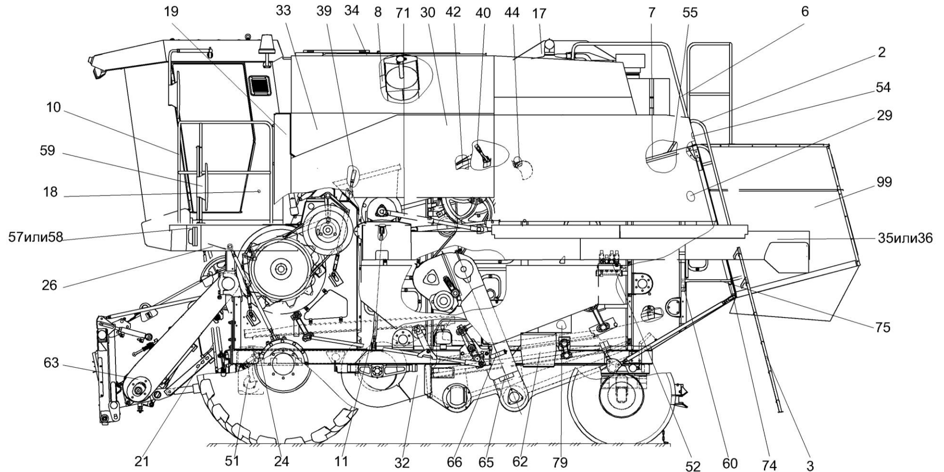
Рисунок 1 – Молотилка самоходная КЗК-10-0100000 (вид слева)
