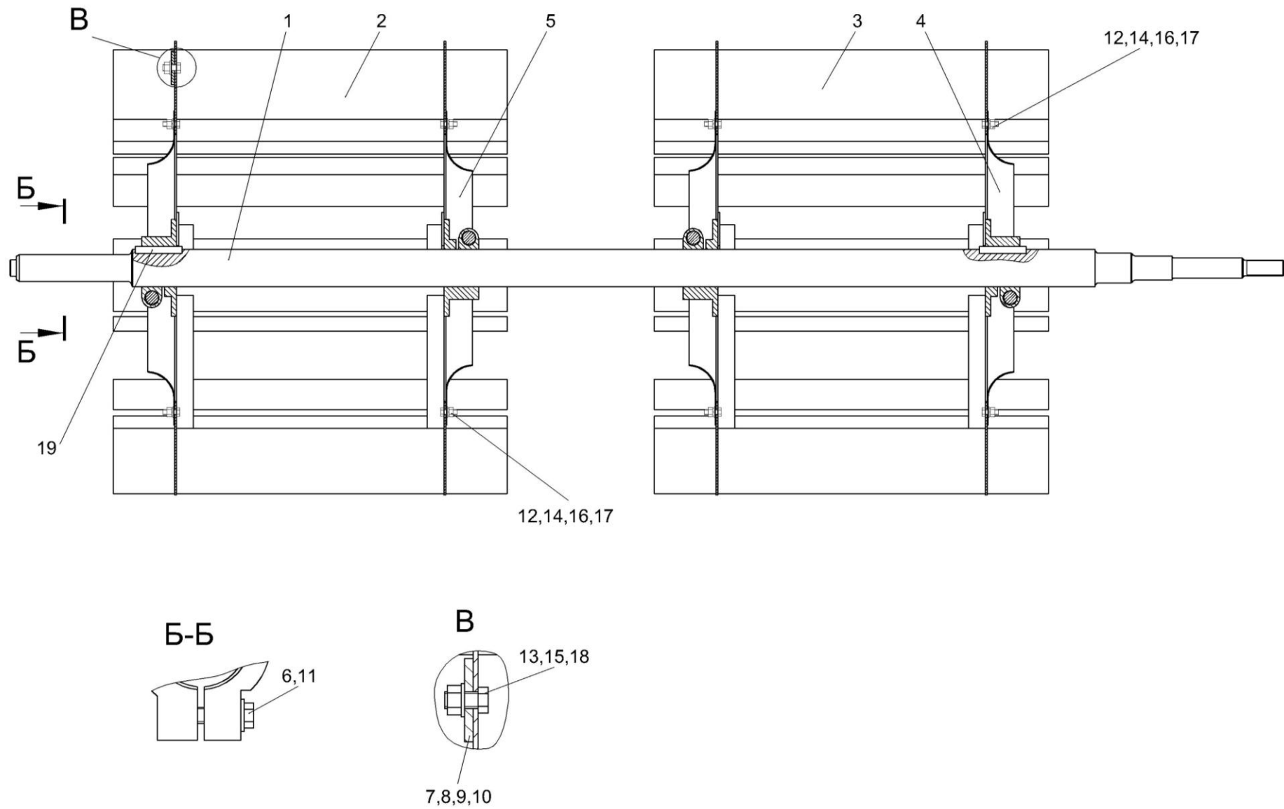
Рисунок 60 – Крылач КЗК-10-0217010
