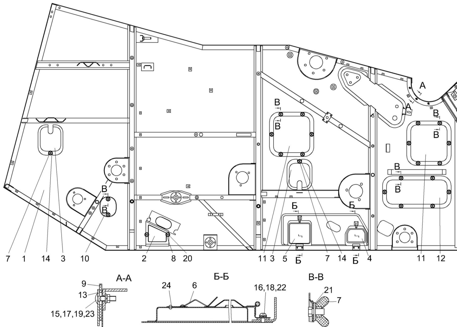
Рисунок 34 – Боковина правая КЗК-10-0202060
