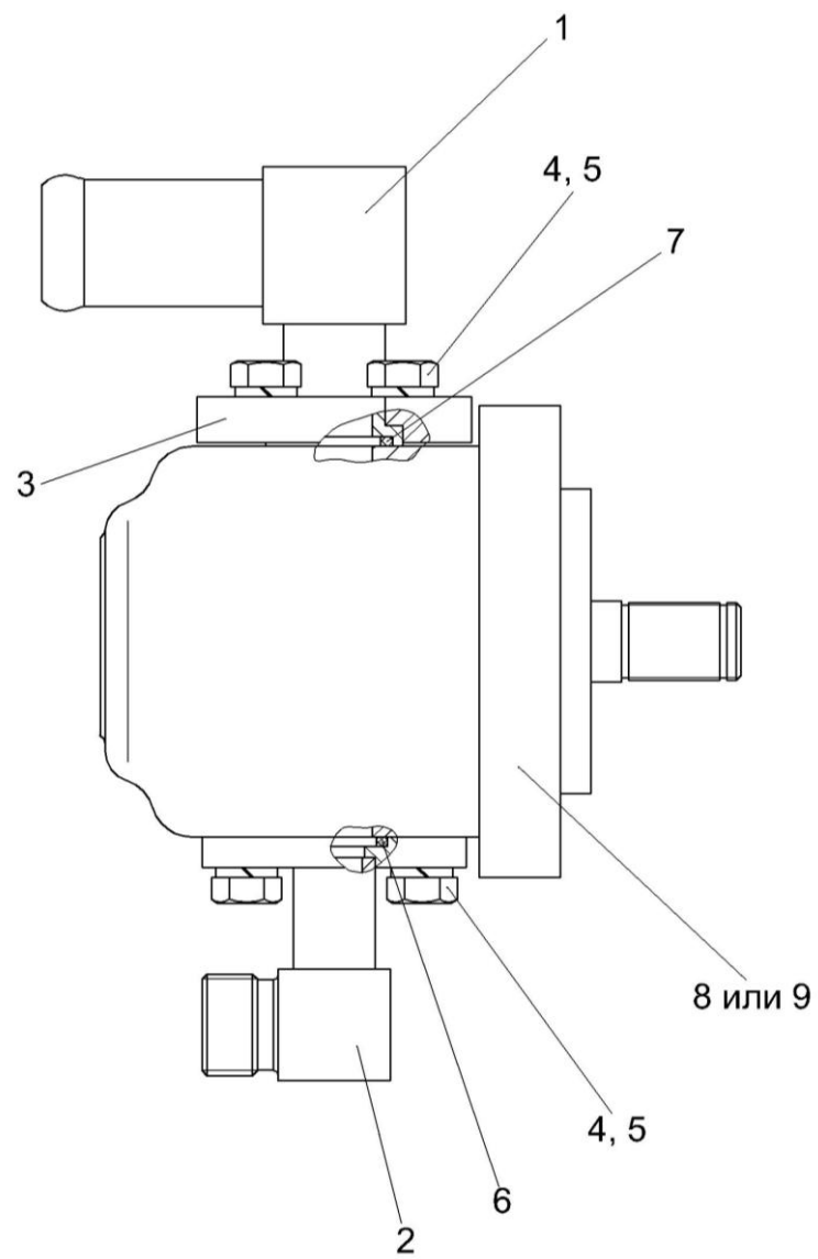
Рисунок 13 – Гидронасос КЗК-10-0602990
