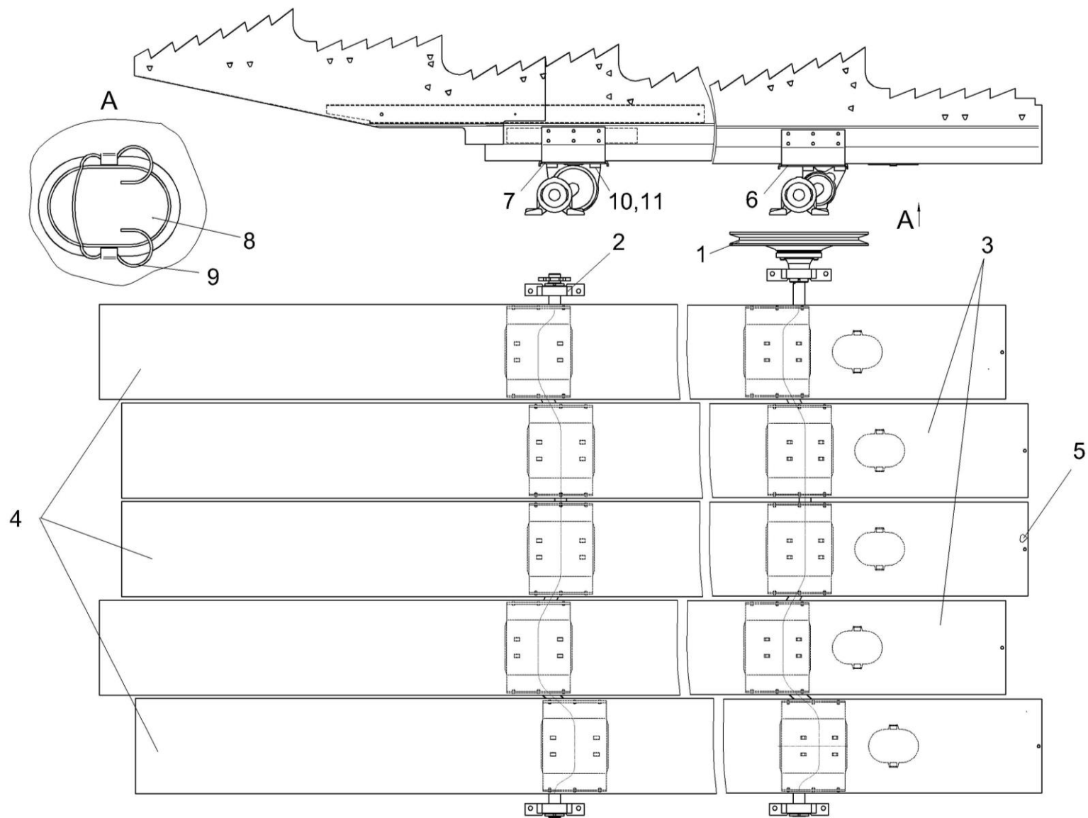
Рисунок 37 – Соломотряс КЗК-10-0212040
