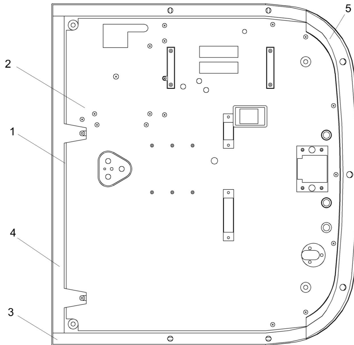
Рисунок 19 – Площадка КЗК-10-0119010
