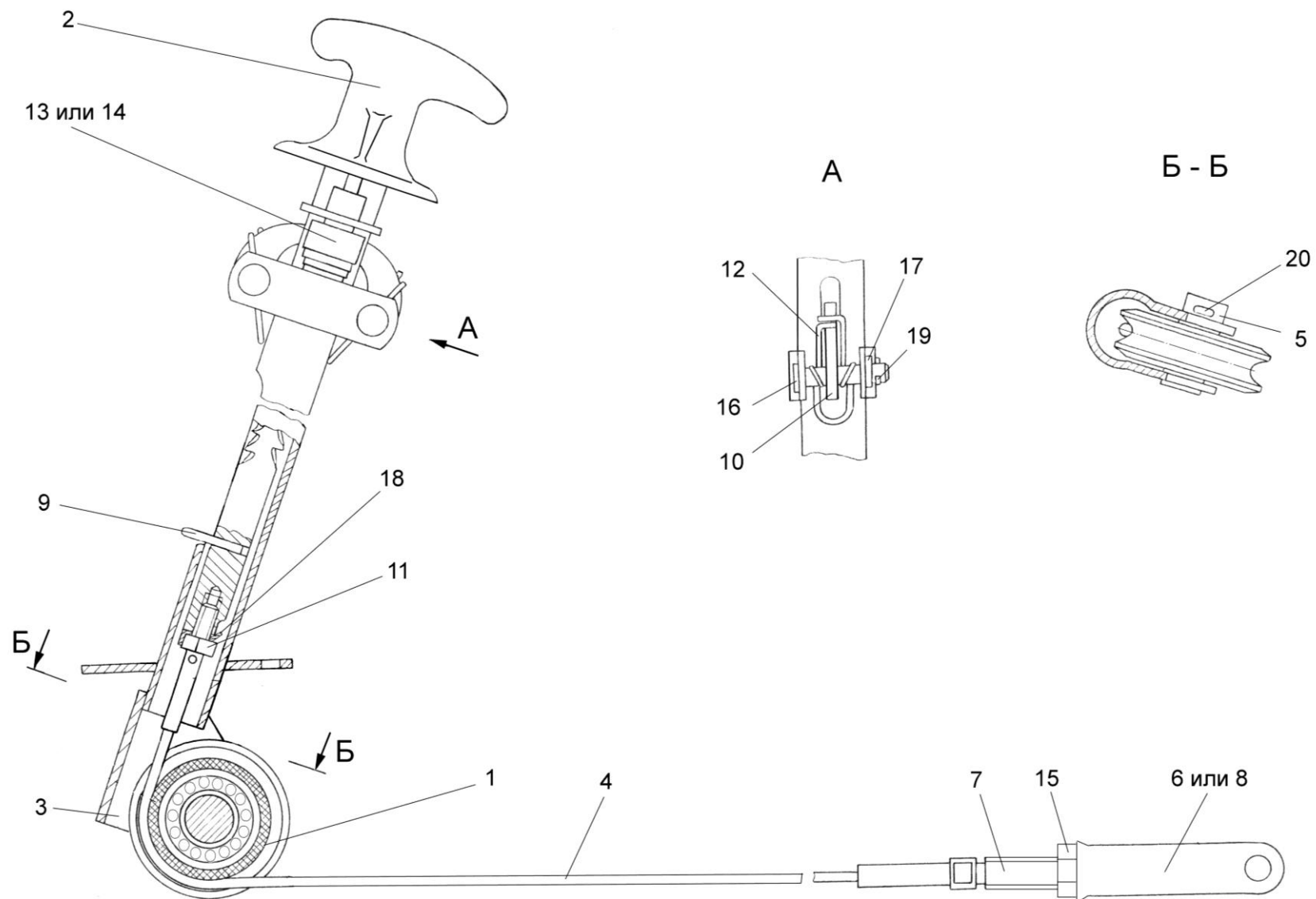
Рисунок 29 – Колонка привода УЭС 0300710
