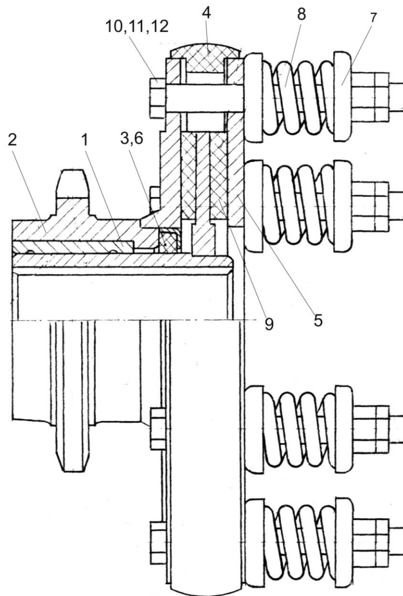
Рисунок 43 – Муфта фрикционная КЗК 0219020Б
