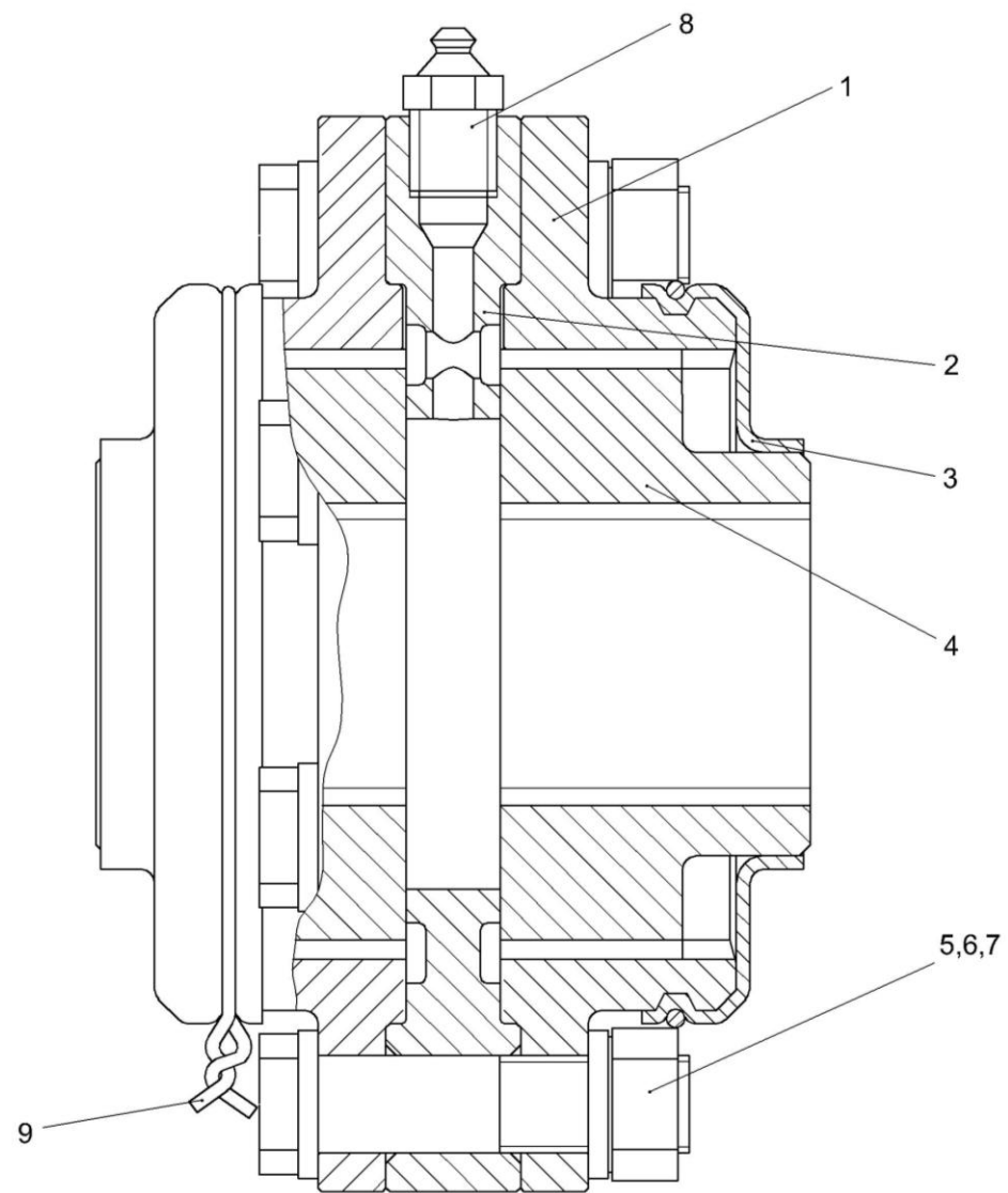
Рисунок 56 – Муфта КЗК-10-0107140
